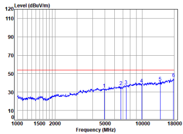
BLE_1M_TX_CH_39_Horizontal-Avg
