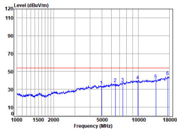
BLE_2M_TX_CH_39_Horizontal-Avg
