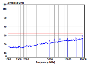
BLE_1M_TX_CH_39_Vertical-Avg
