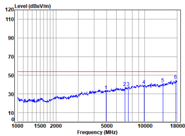
BLE_2M_TX_CH_39_Vertical-Avg
