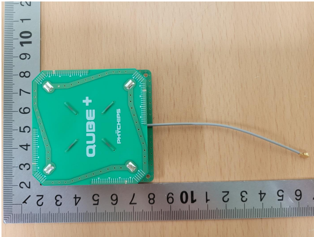
Antenna 1 (M/N: QUBE 6015 PLUS)
