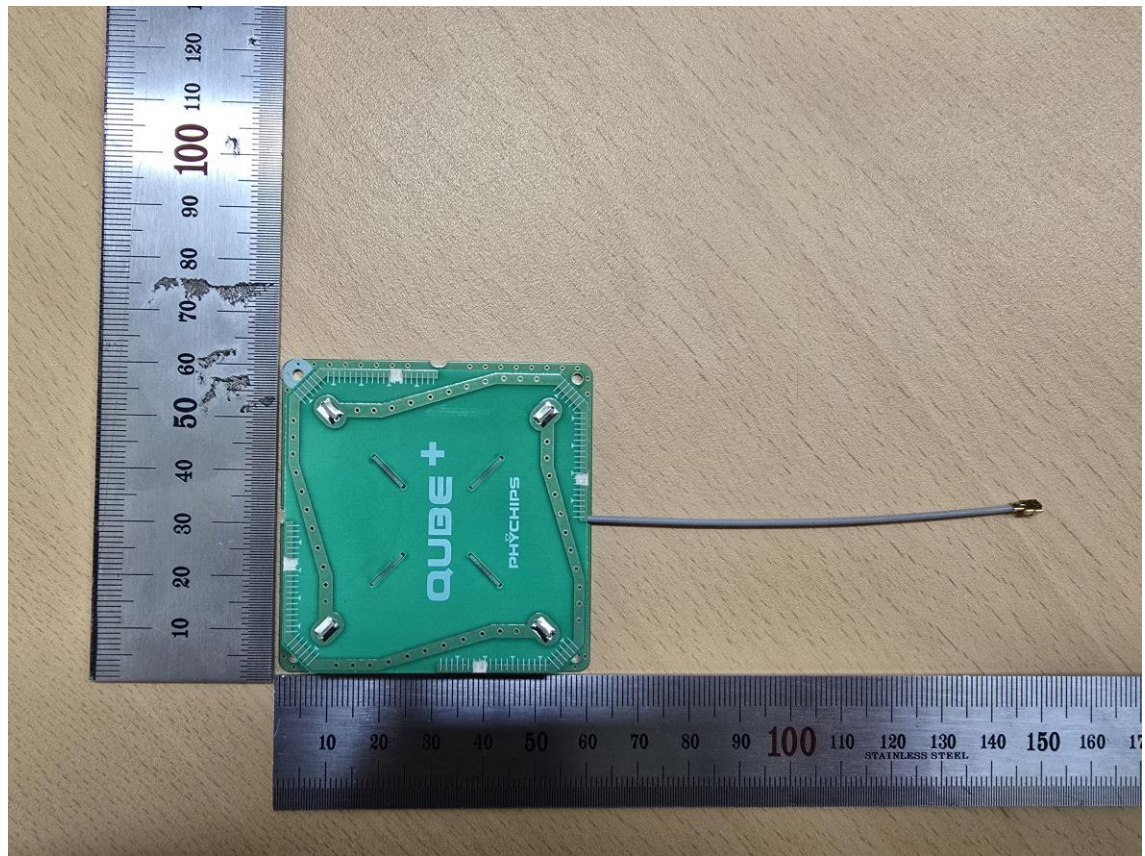
Antenna 5 (M/N: QUBE 6010 PLUS)
