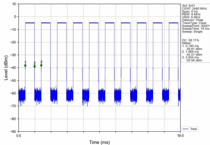
2M_HCH_2480MHz_Ant1_NTNV
