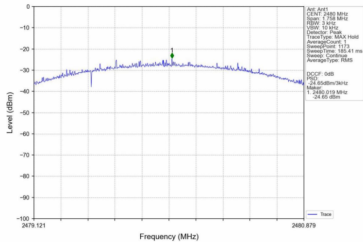
2M_HCH_2480MHz_Ant1_NTNV
