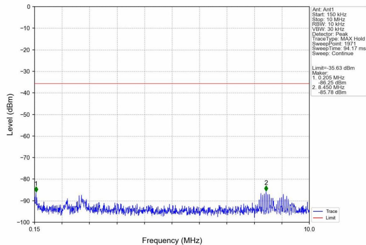
2M_HCH_2480MHz_Ant1_NTNV
