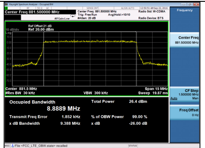
OBW- Band5-10M BW-Mid
