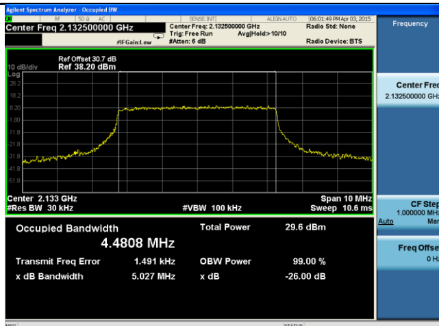
OBW-Band4-5M BW-Mid
