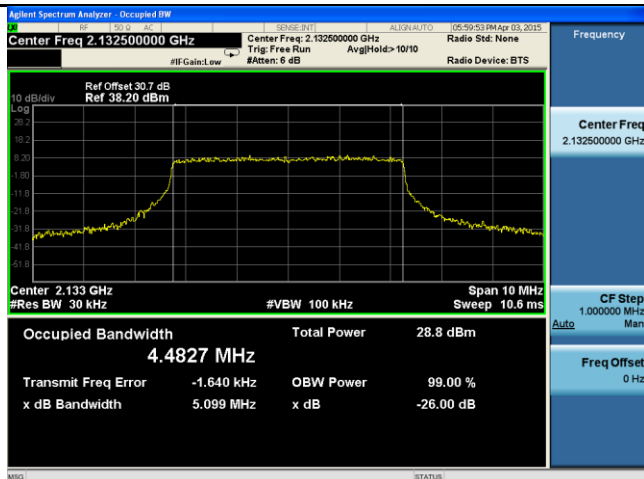
OBW-Band4-5M BW-Mid
