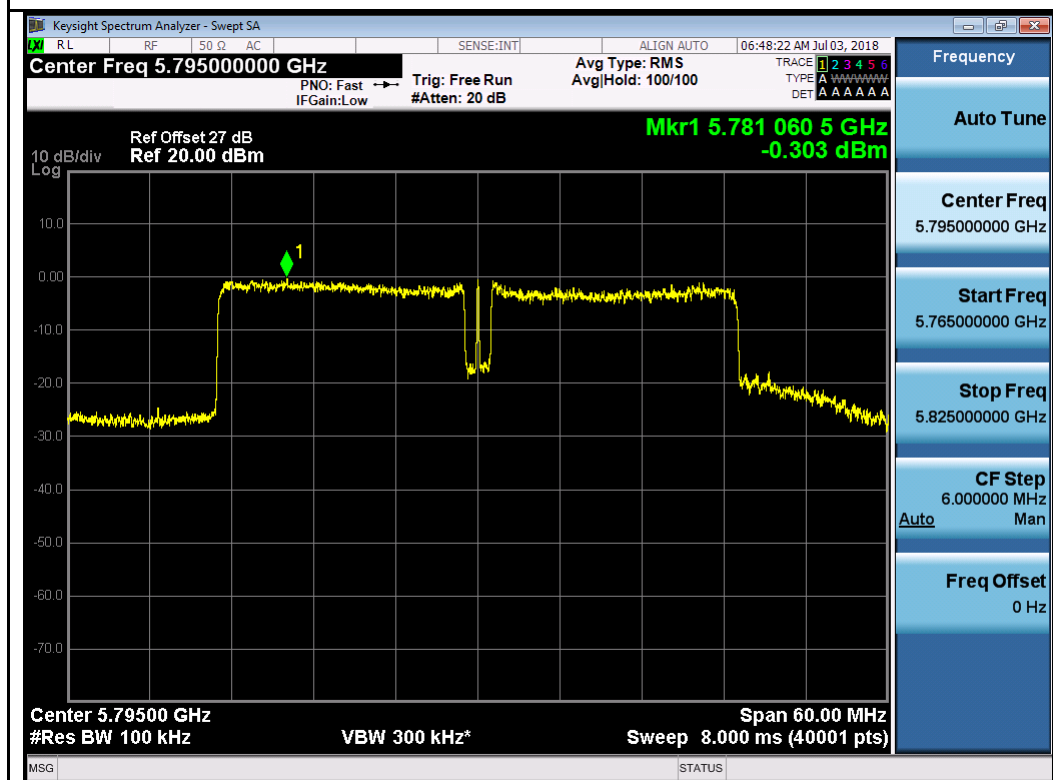
QPSK-5795MHz
