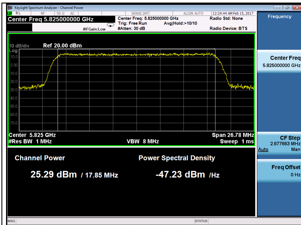
QPSK-5825MHz
