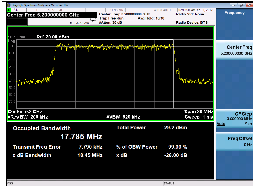
QPSK-5200MHz
