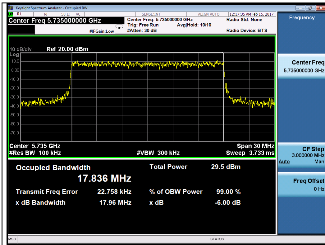
QPSK-5735MHz
