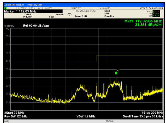
30-200 MHz Horizontal
