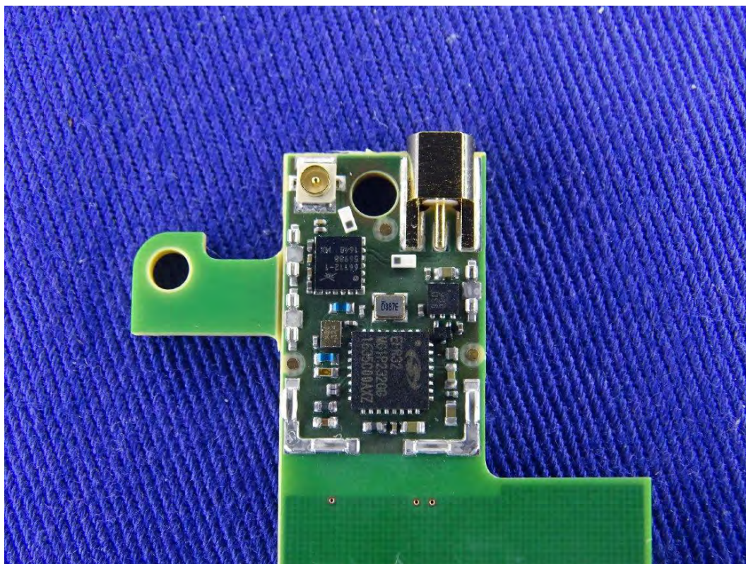
(4) EUT Photo (M/N: EMIP400)
