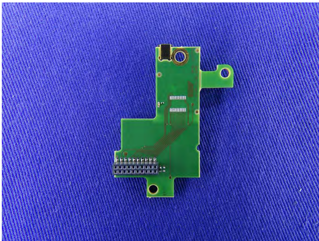
(5) EUT Photo (M/N: EMIP400)
