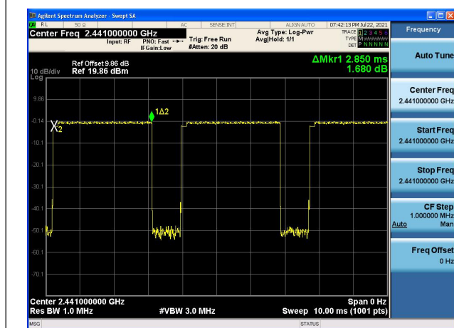
Modulation: \pi/4 DQPSK 2DH5 2441
