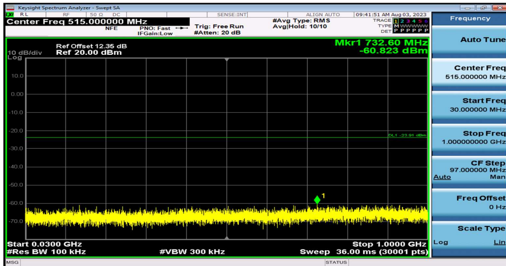
11G_Ant1_2412_30~1000
