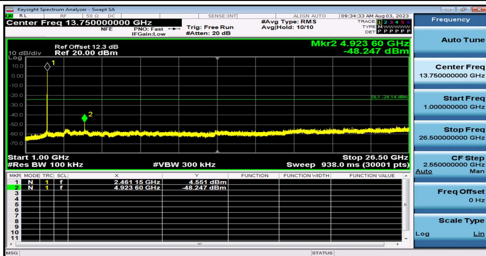
11B_Ant1_2462_1000~26500
