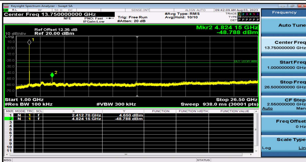
11G_Ant1_2412_1000~26500
