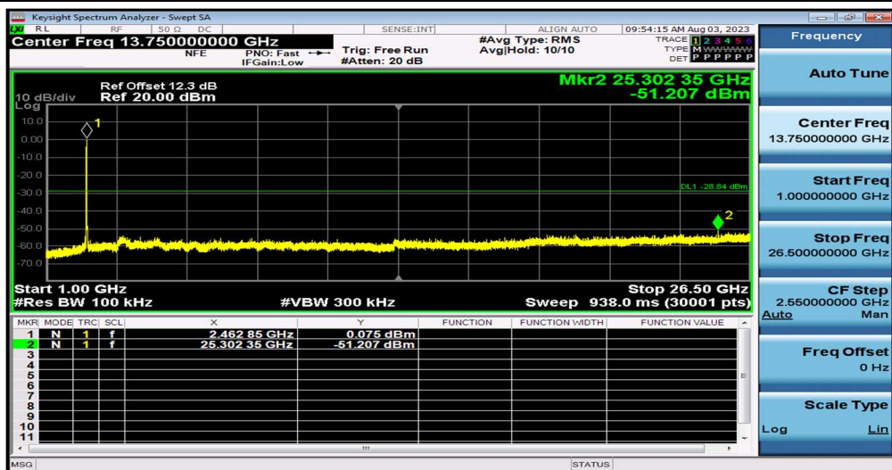
11G_Ant1_2462_1000~26500
