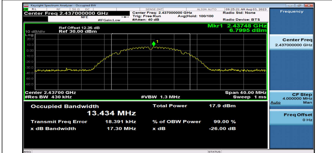
11B_Ant1_2437
