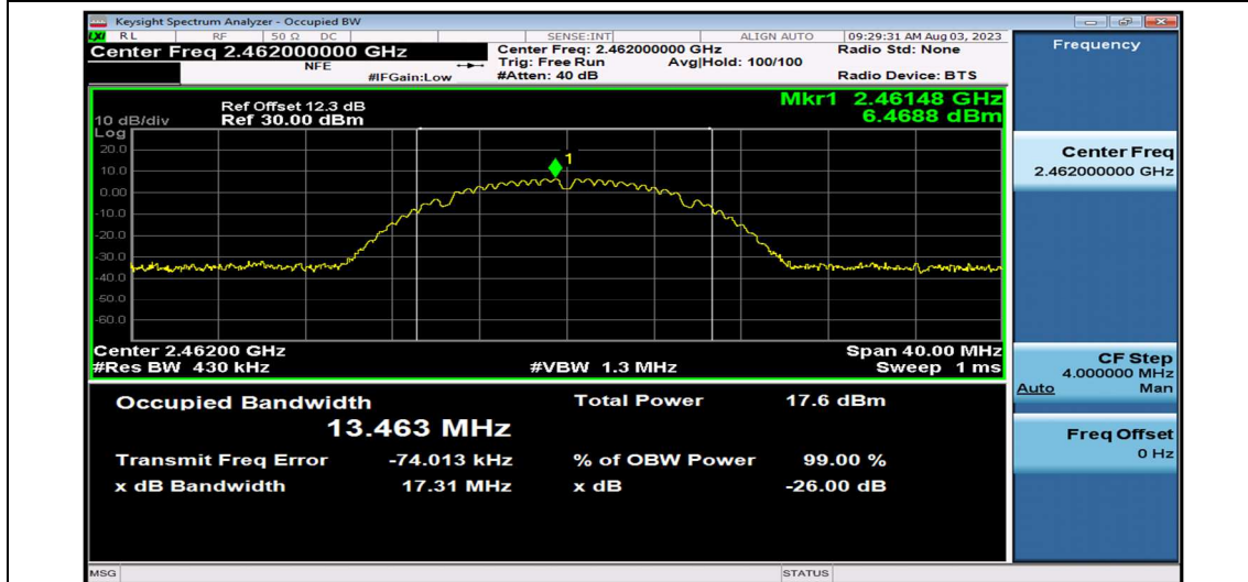
11B_Ant1_2462
