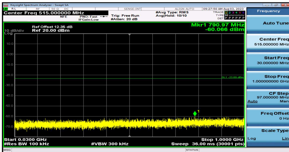
11B_Ant1_2437_30~1000
