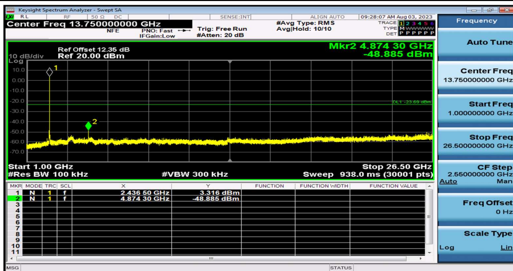
11B_Ant1_2437_1000~26500
