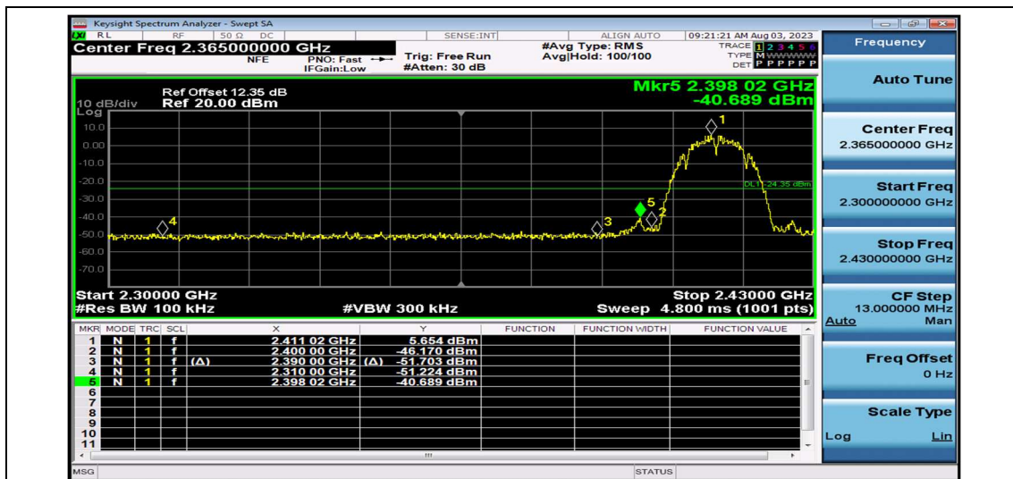
11B_Ant1_Low_2412
