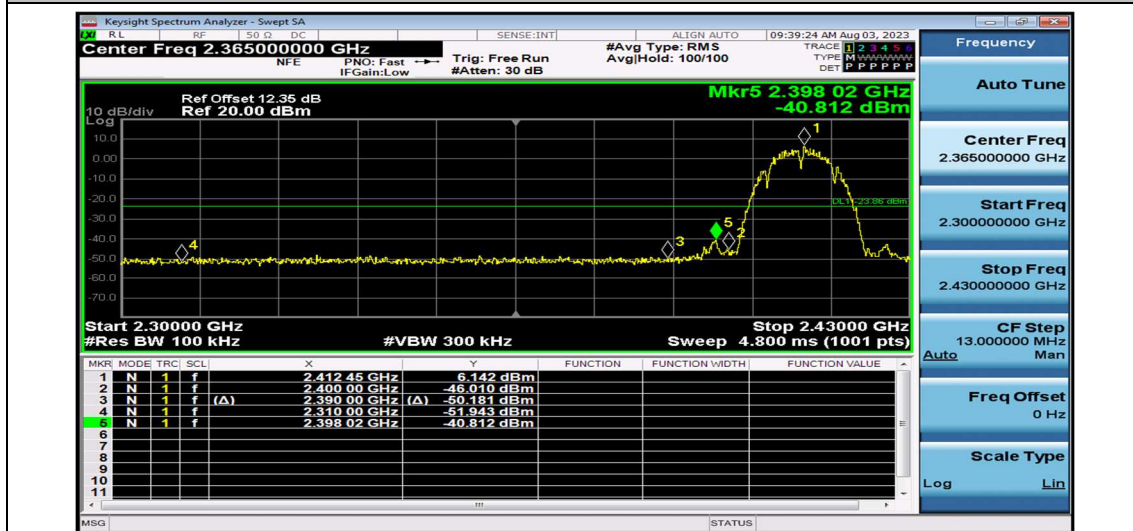
11G_Ant1_Low_2412
