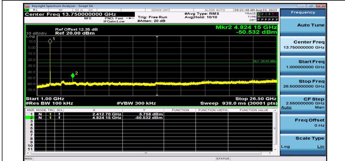
11B_Ant1_2412_1000~26500
