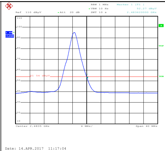
Band Edge, Right Side (Average - Horizontal)
