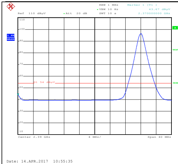
Band Edge, Left Side (Average - Horizontal)
