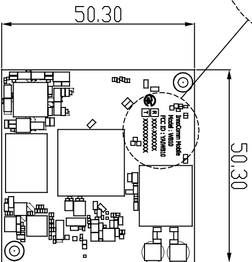
TOP SIDE
