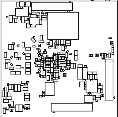
BOTTOM SIDE
