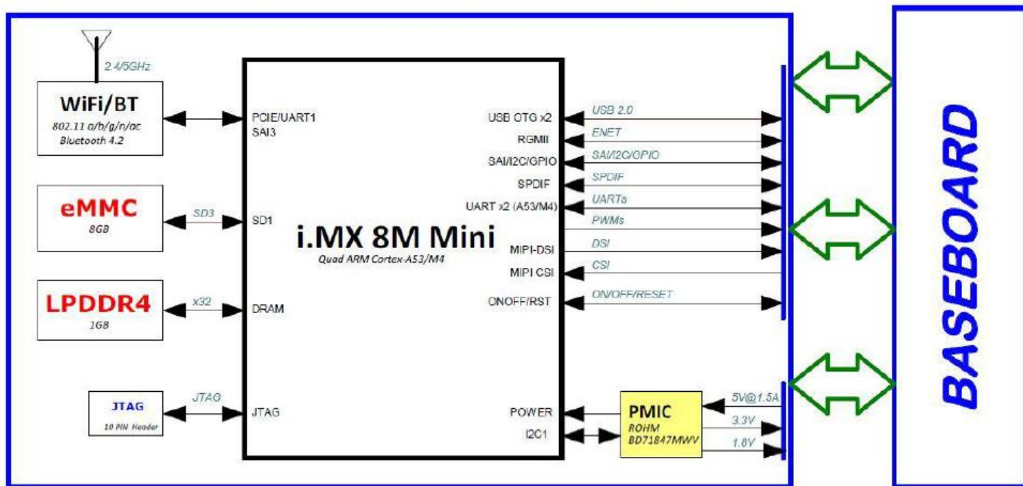
Figure 1-1 WB15 SOM Block Diagram
