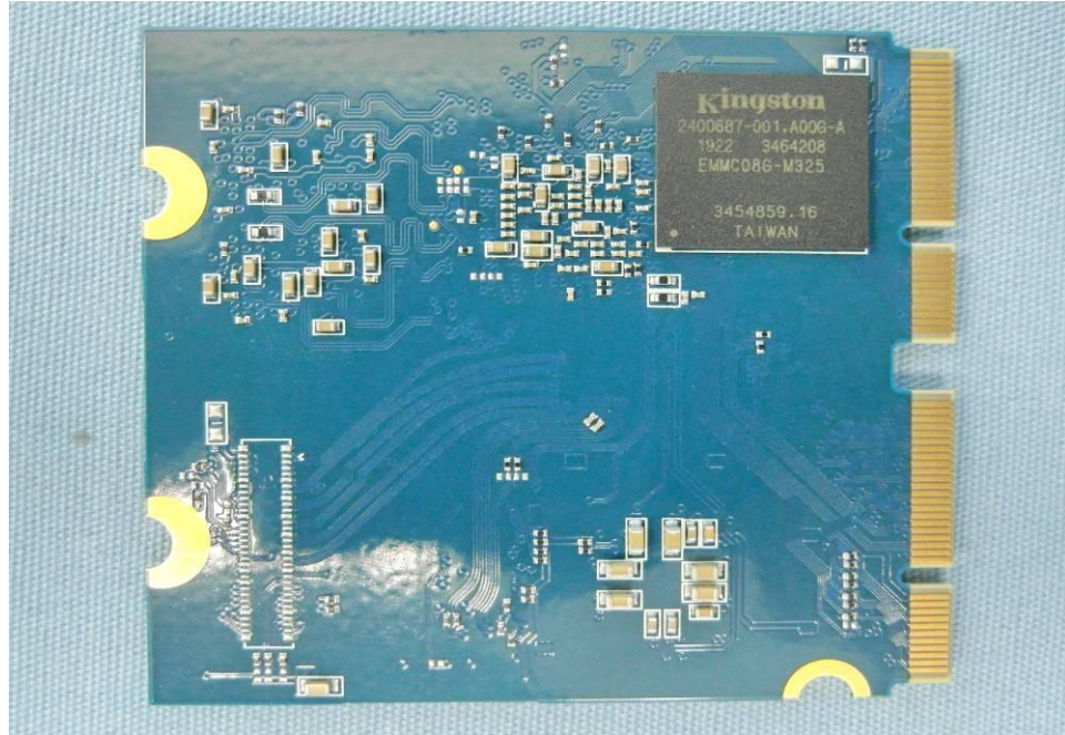
EUT Photo (3)
