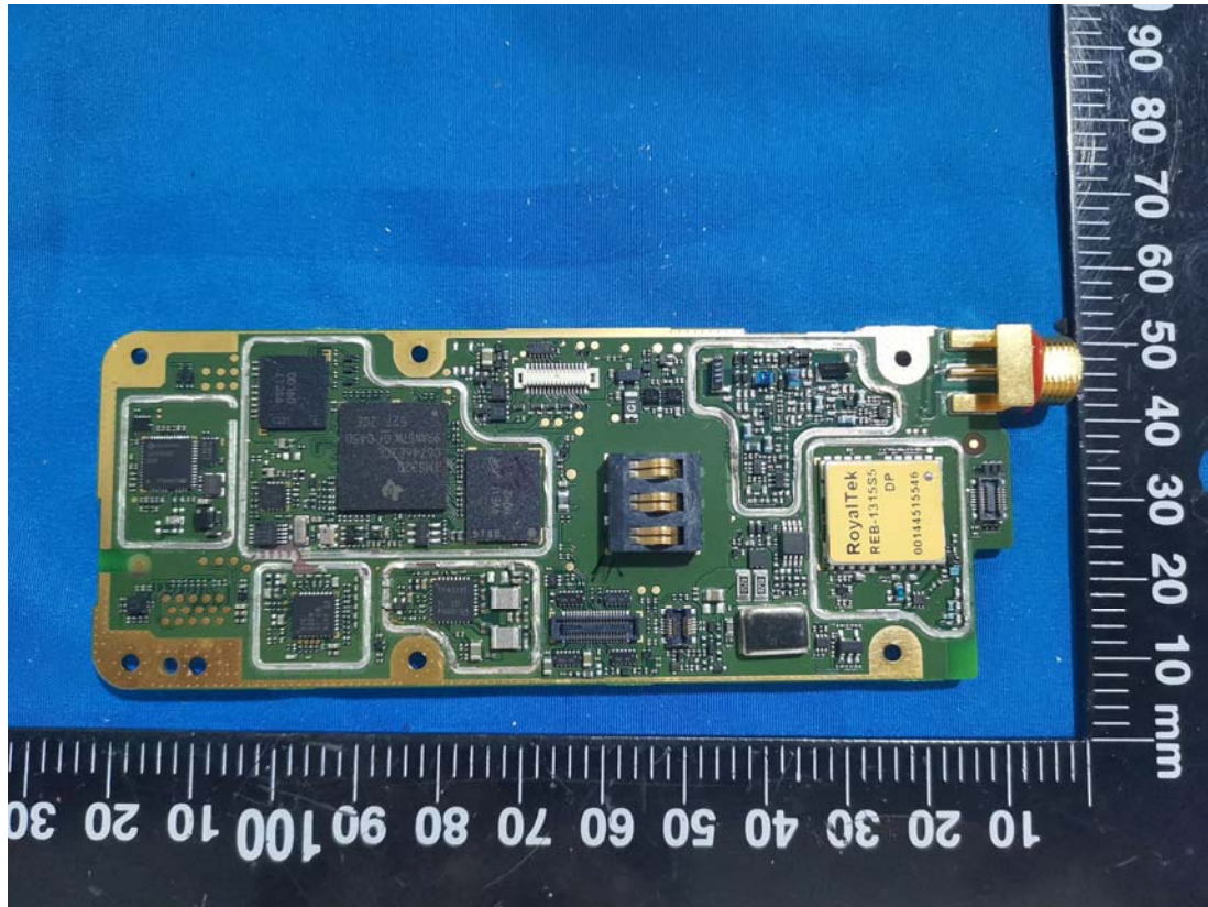
GPS Module
