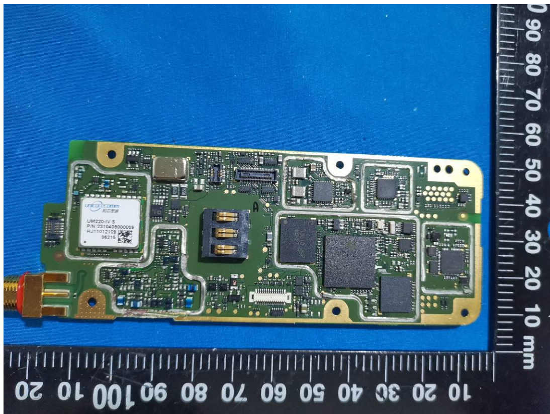
GPS Module
