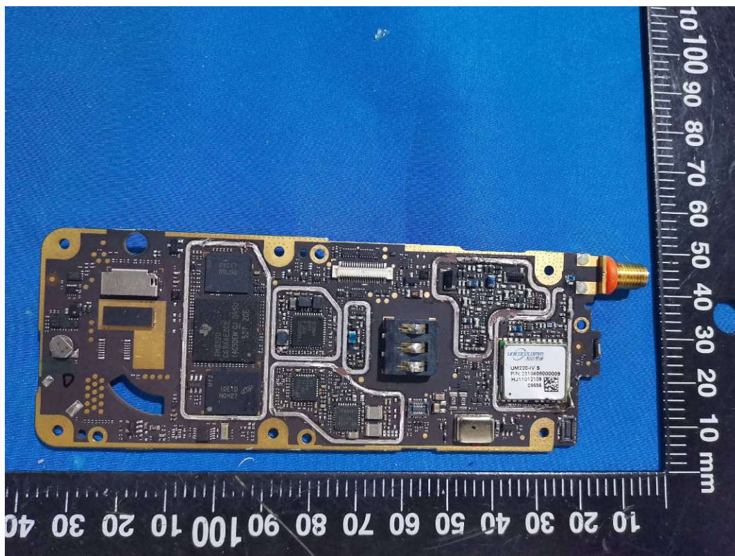
GPS Module
