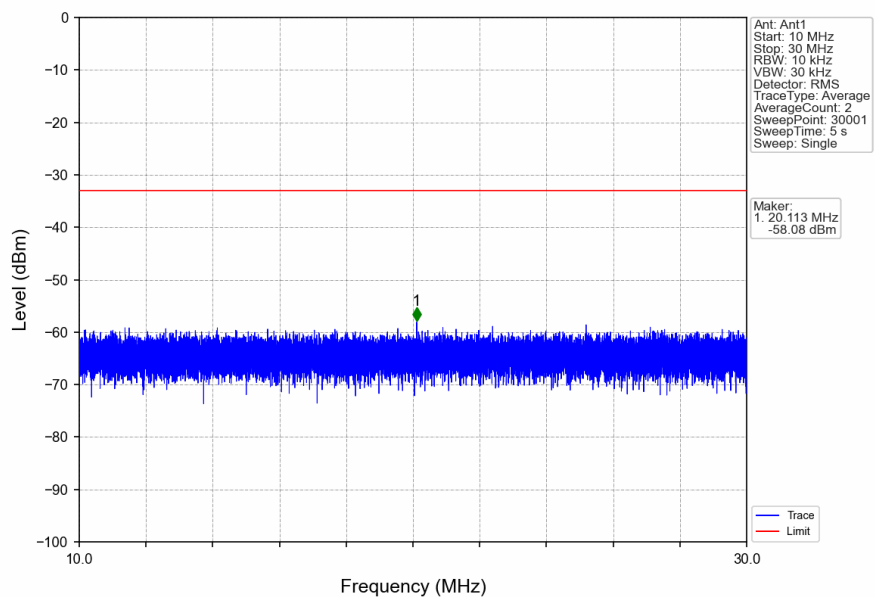
n2_15kHz_SISO_NTNV_5MHz_CP-OFDM_QPSK_1852.5MHz_Inner_1RB_Left
