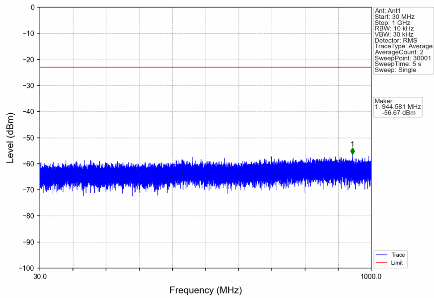
n2_15kHz_SISO_NTNV_5MHz_CP-OFDM QPSK_1880MHz_Edge_1RB_Left
