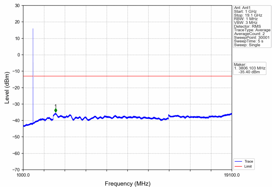
n2_15kHz_SISO_NTNV_5MHz_CP-OFDM_QPSK_1852.5MHz_Inner_1RB_Left
