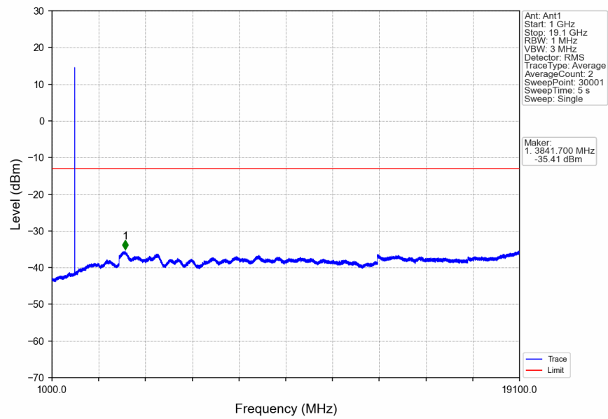
n2_15kHz_SISO_NTNV_5MHz_CP-OFDM QPSK_1880MHz_Edge_1RB_Left
