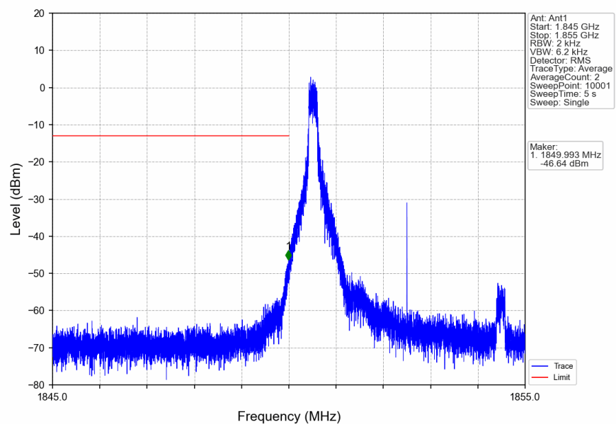
n2_15kHz_SISO_NTNV_5MHz_CP-OFDM_QPSK_1852.5MHz_Inner_1RB_Left
