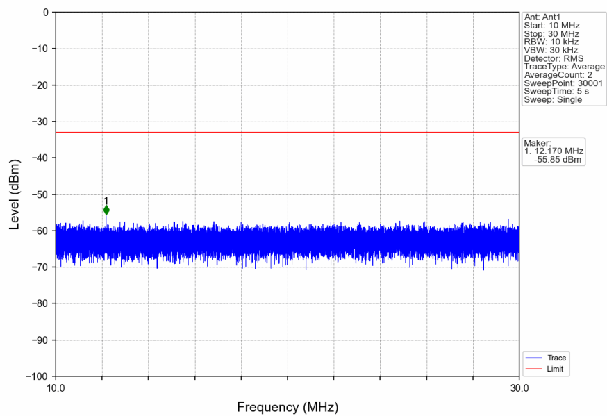
n2_15kHz_SISO_NTNV_5MHz_DFT-s-OFDM PI/2 BPSK_1880MHz_Edge_1RB_Left
