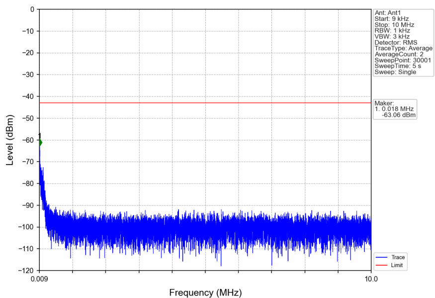
n2_15kHz_SISO_NTNV_5MHz_CP-OFDM_QPSK_1852.5MHz_Inner_1RB_Left
