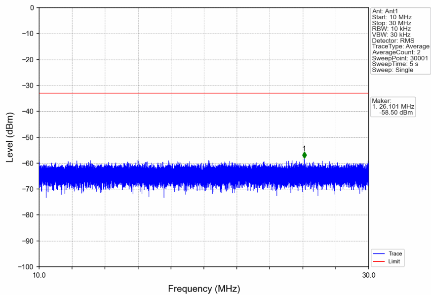
n2_15kHz_SISO_NTNV_10MHz_DFT-s-OFDM_QPSK_1855MHz_Inner_1RB_Left
