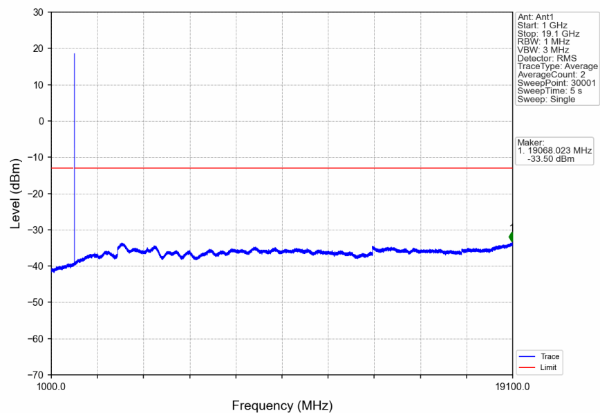
n2_15kHz_SISO_NTNV_10MHz_DFT-s-OFDM PI/2 BPSK_1905MHz_Inner_1RB_Right
