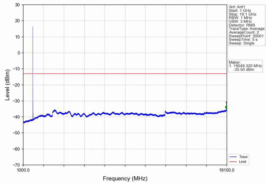
n2_15kHz_SISO_NTNV_10MHz_DFT-s-OFDM_QPSK_1855MHz_Inner_1RB_Left
