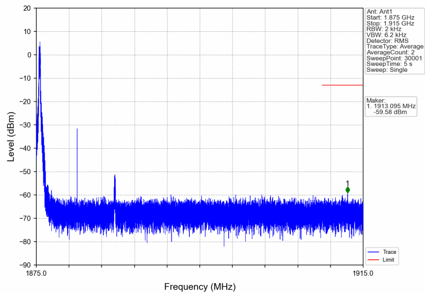
n2_15kHz_SISO_NTNV_10MHz_DFT-s-OFDM PI/2 BPSK_1880MHz_Edge_1RB_Left
