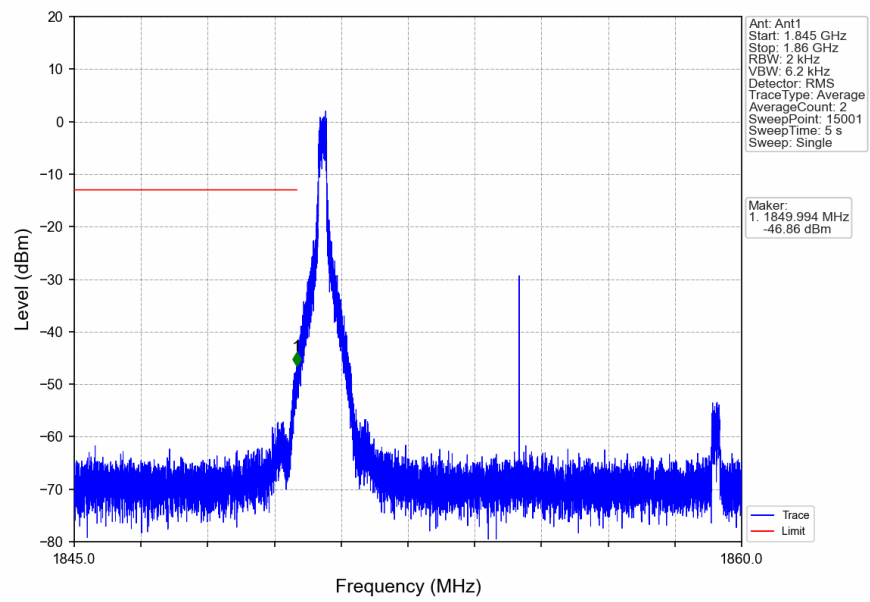
n2_15kHz_SISO_NTNV_10MHz_CP-OFDM_QPSK_1855MHz_Inner_1RB_Left
