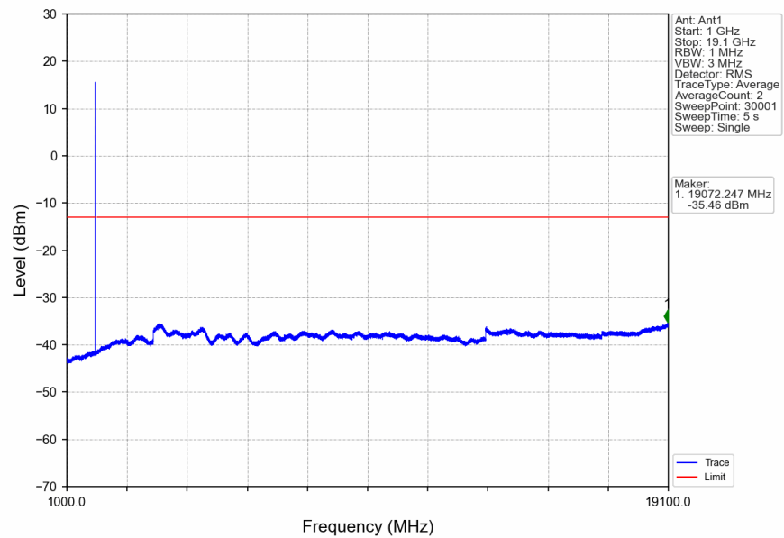
n2_15kHz_SISO_NTNV_10MHz_CP-OFDM_QPSK_1855MHz_Inner_1RB_Left
