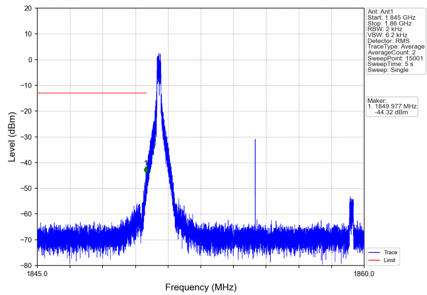
n2_15kHz_SISO_NTNV_10MHz_DFT-s-OFDM_QPSK_1855MHz_Inner_1RB_Left
