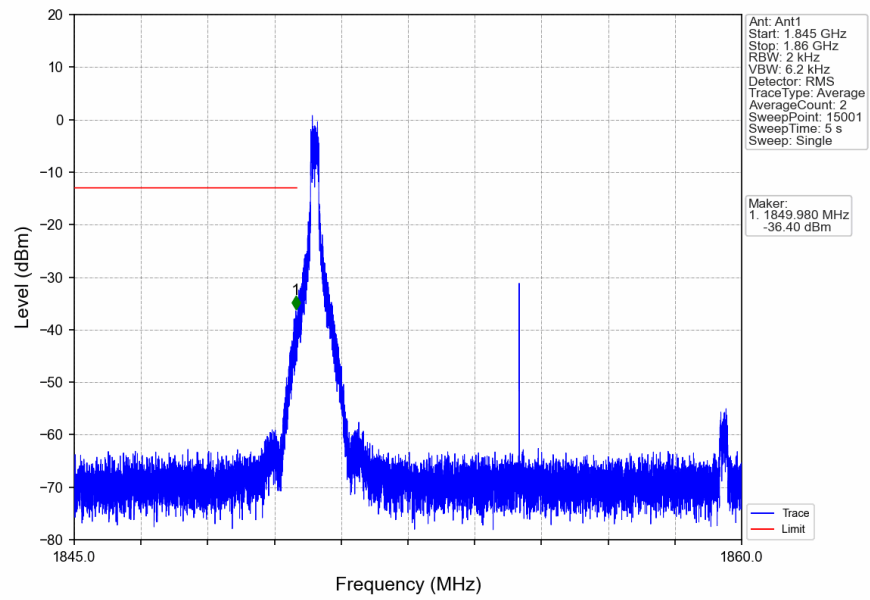
n2_15kHz_SISO_NTNV_10MHz_CP-OFDM_QPSK_1855MHz_Edge_1RB_Left
