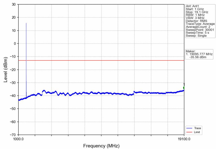
n2_15kHz_SISO_NTNV_10MHz_DFT-s-OFDM_QPSK_1855MHz_Edge_1RB_Left
