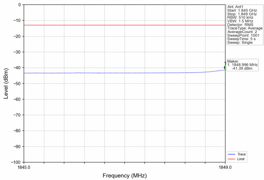
n2_15kHz_SISO_NTNV_10MHz_DFT-s-OFDM_PI/2_BPSK_1855MHz_Inner_1RB_Left
