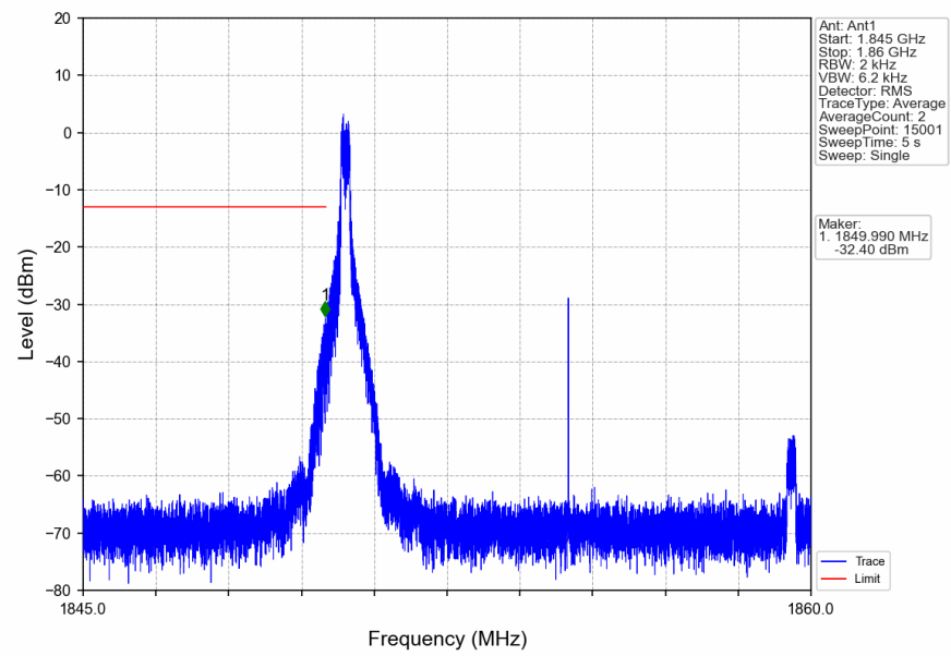
n2_15kHz_SISO_NTNV_10MHz_DFT-s-OFDM_QPSK_1855MHz_Edge_1RB_Left
