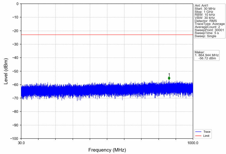
n2_15kHz_SISO_NTNV_10MHz_DFT-s-OFDM_QPSK_1855MHz_Inner_1RB_Left
