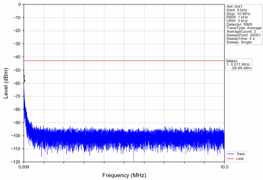
n2_15kHz_SISO_NTNV_10MHz_CP-OFDM_QPSK_1855MHz_Edge_1RB_Left
