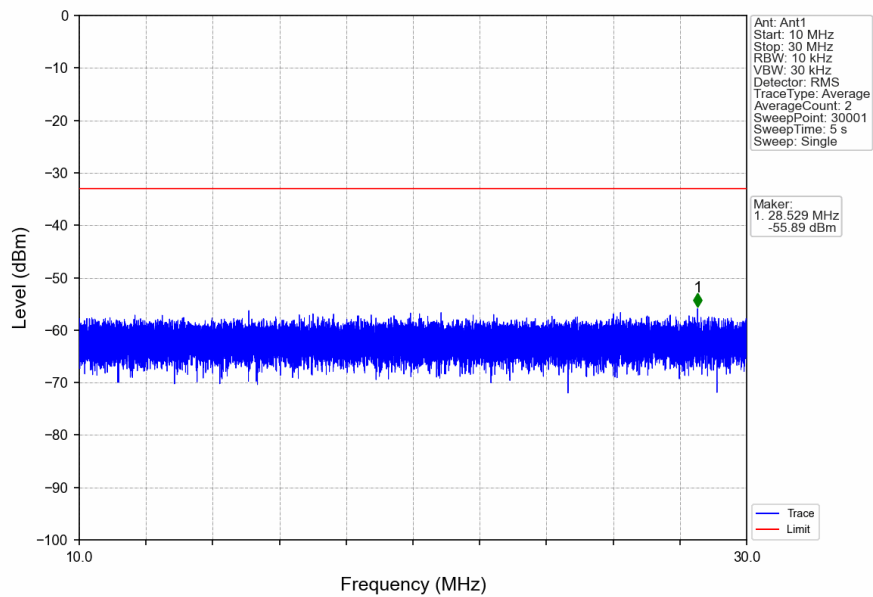
n2_15kHz_SISO_NTNV_10MHz_DFT-s-OFDM PI/2 BPSK_1880MHz_Edge_1RB_Left
