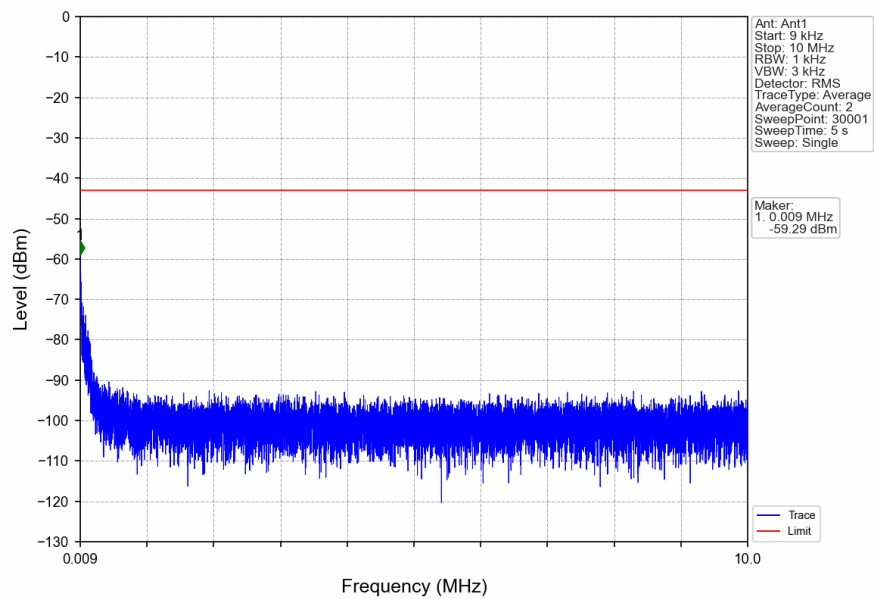
n2_15kHz_SISO_NTNV_10MHz_DFT-s-OFDM_QPSK_1855MHz_Edge_1RB_Left
