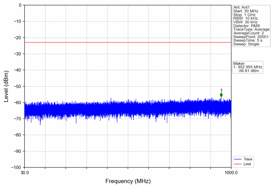
n2_15kHz_SISO_NTNV_10MHz_DFT-s-OFDM_QPSK_1855MHz_Edge_1RB_Left
