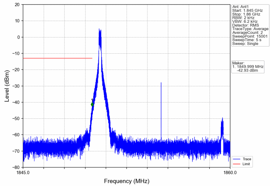
n2_15kHz_SISO_NTNV_10MHz_DFT-s-OFDM_PI/2_BPSK_1855MHz_Inner_1RB_Left
