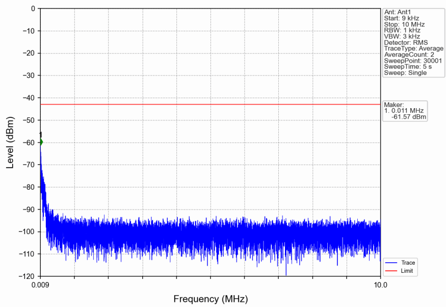
n2_15kHz_SISO_NTNV_10MHz_CP-OFDM QPSK_1905MHz_Inner_1RB_Right
