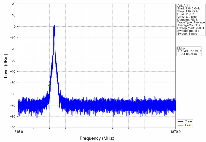
n2_15kHz_SISO_NTNV_20MHz_DFT-s-OFDM_QPSK_1860MHz_Inner_1RB_Left
