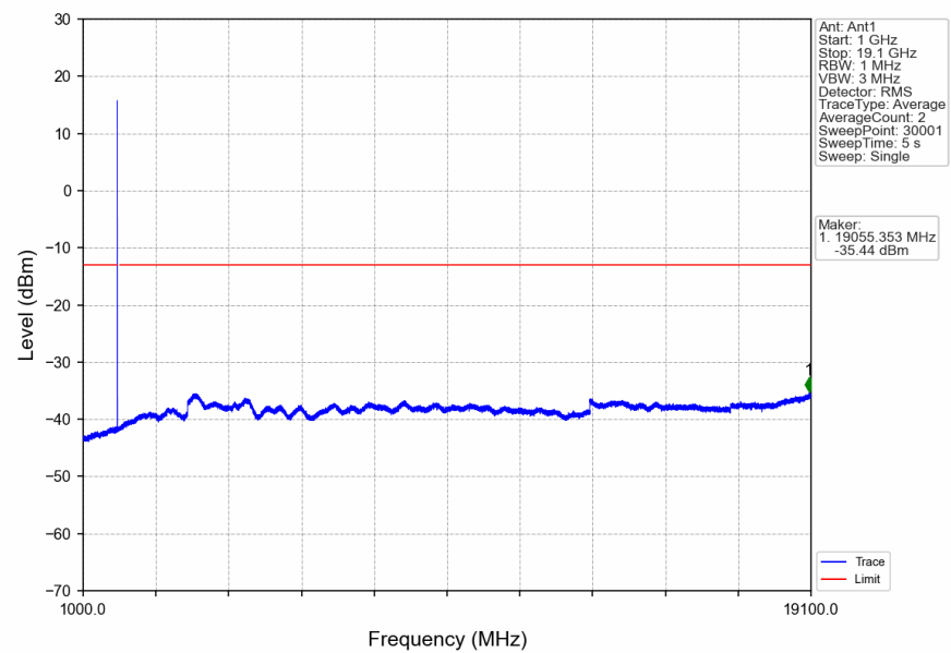
n2_15kHz_SISO_NTNV_20MHz_DFT-s-OFDM_QPSK_1860MHz_Edge_1RB_Left
