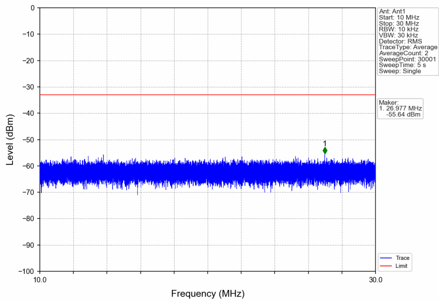
n2_15kHz_SISO_NTNV_20MHz_DFT-s-OFDM PI/2 BPSK_1860MHz_Edge_1RB_Left
