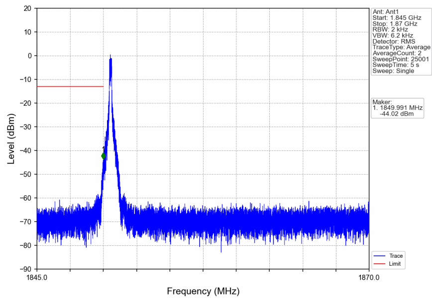
n2_15kHz_SISO_NTNV_20MHz_CP-OFDM_QPSK_1860MHz_Edge_1RB_Left
