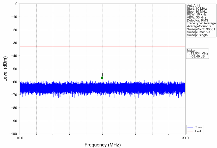
n2_15kHz_SISO_NTNV_20MHz_DFT-s-OFDM_QPSK_1900MHz_Inner_1RB_Right
