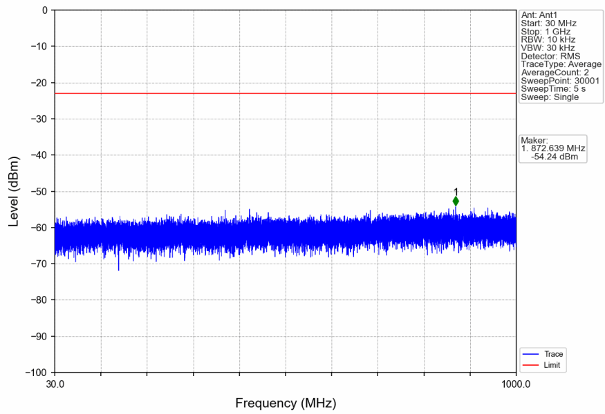
n2_15kHz_SISO_NTNV_20MHz_DFT-s-OFDM PI/2 BPSK_1860MHz_Inner_1RB_Left
