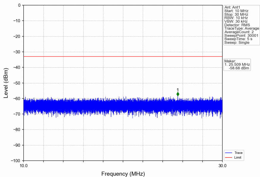
n2_15kHz_SISO_NTNV_20MHz_DFT-s-OFDM_QPSK_1860MHz_Edge_1RB_Left
