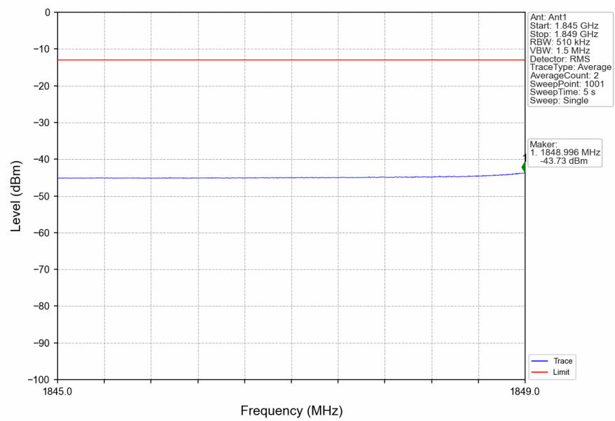
n2_15kHz_SISO_NTNV_20MHz_DFT-s-OFDM_QPSK_1860MHz_Inner_1RB_Left
