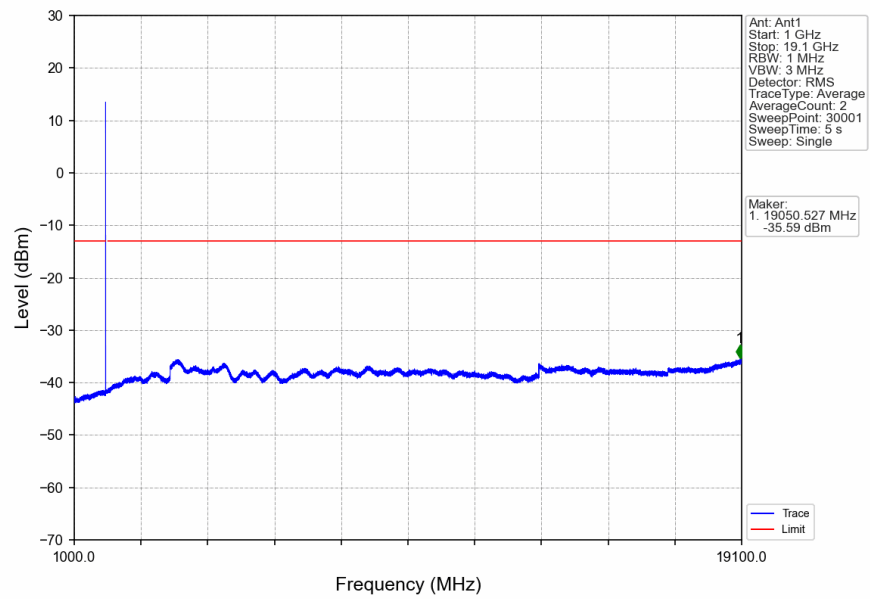
n2_15kHz_SISO_NTNV_20MHz_CP-OFDM_QPSK_1860MHz_Edge_1RB_Left
