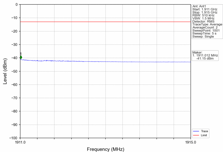
n2_15kHz_SISO_NTNV_20MHz_DFT-s-OFDM PI/2 BPSK_1900MHz_Inner_1RB_Right
