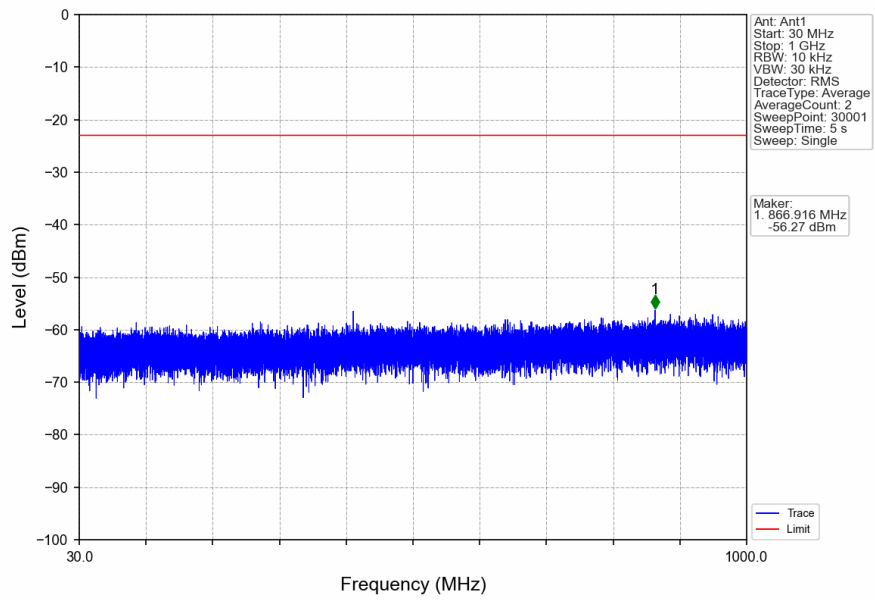
n2_15kHz_SISO_NTNV_20MHz_CP-OFDM_QPSK_1860MHz_Edge_1RB_Left
