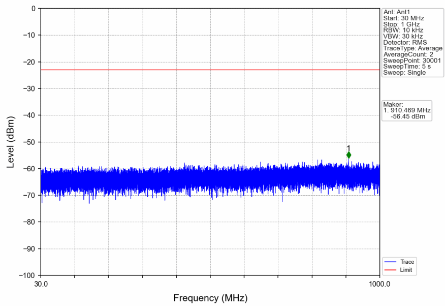
n2_15kHz_SISO_NTNV_20MHz_DFT-s-OFDM_QPSK_1900MHz_Inner_1RB_Right
