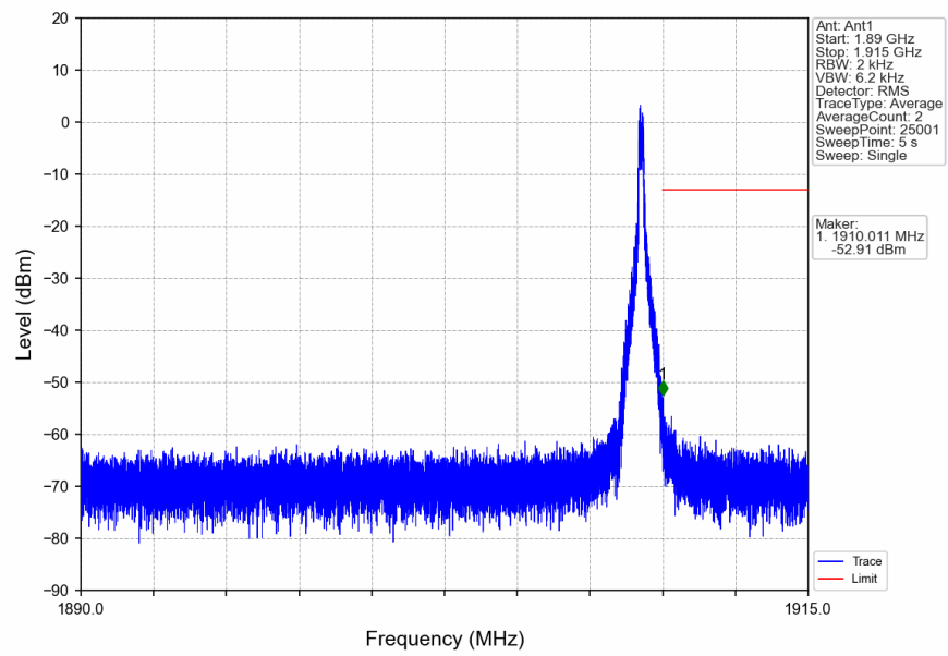
n2_15kHz_SISO_NTNV_20MHz_DFT-s-OFDM_QPSK_1900MHz_Inner_1RB_Right
