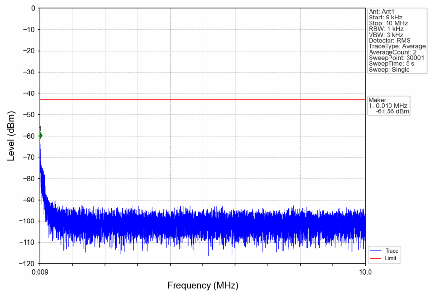
n2_15kHz_SISO_NTNV_20MHz_DFT-s-OFDM_QPSK_1860MHz_Inner_1RB_Left
