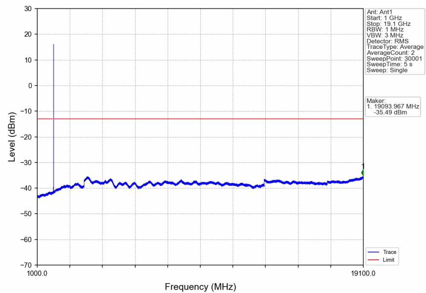
n2_15kHz_SISO_NTNV_20MHz_DFT-s-OFDM_QPSK_1900MHz_Inner_1RB_Right
