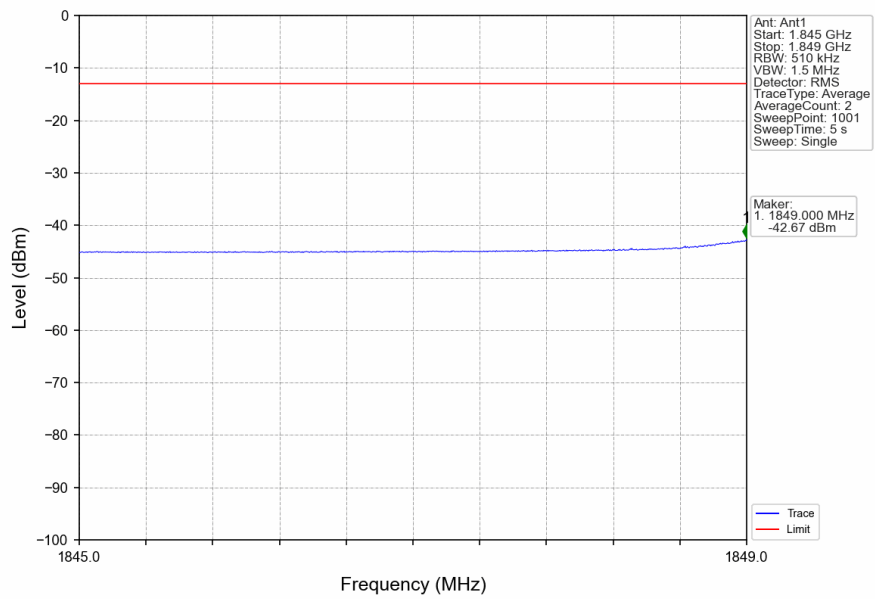
n2_15kHz_SISO_NTNV_20MHz_DFT-s-OFDM_QPSK_1860MHz_Edge_1RB_Left
