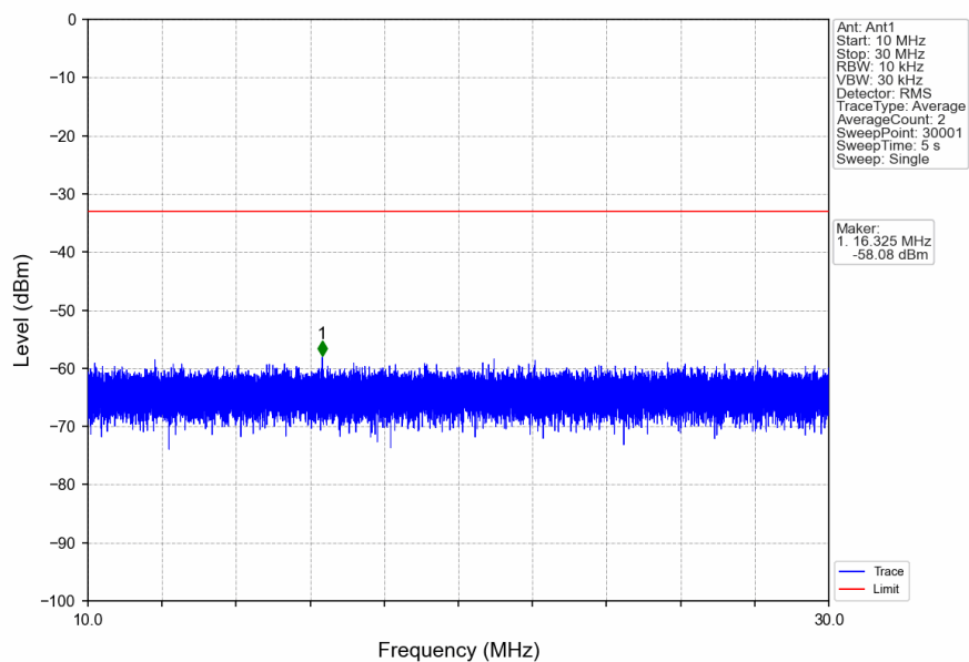
n2_15kHz_SISO_NTNV_20MHz_DFT-s-OFDM_QPSK_1880MHz_Edge_1RB_Left
