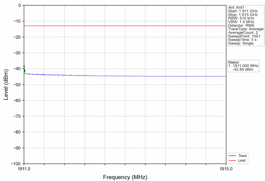
n2_15kHz_SISO_NTNV_20MHz_DFT-s-OFDM_QPSK_1900MHz_Inner_1RB_Right
