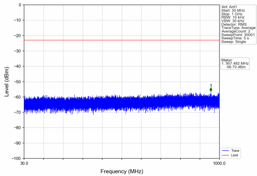
n2_15kHz_SISO_NTNV_20MHz_DFT-s-OFDM_QPSK_1860MHz_Edge_1RB_Left
