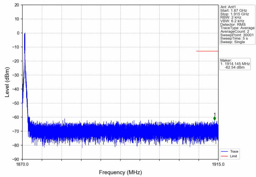
n2_15kHz_SISO_NTNV_20MHz_CP-OFDM_QPSK_1880MHz_Edge_1RB_Left
