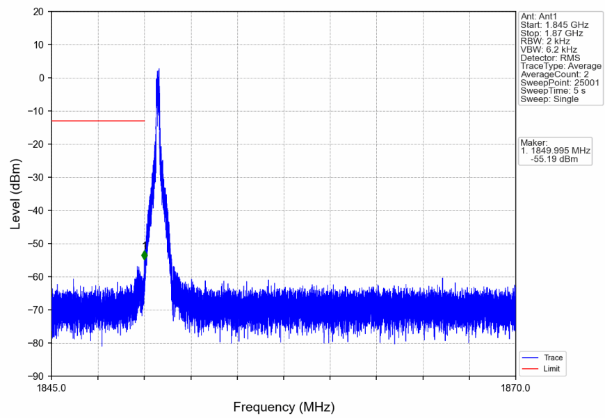
n2_15kHz_SISO_NTNV_20MHz_CP-OFDM_QPSK_1860MHz_Inner_1RB_Left
