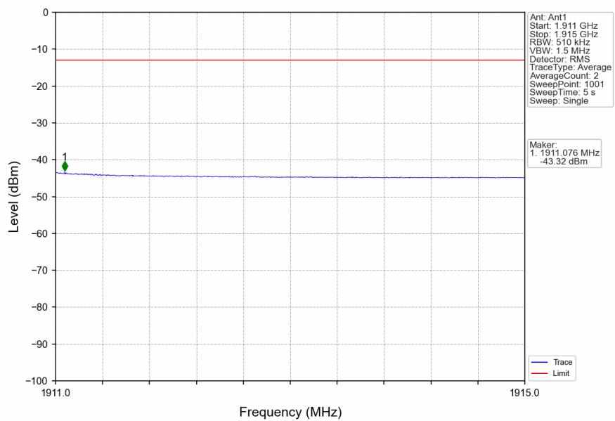
n2_15kHz_SISO_NTNV_20MHz_CP-OFDM QPSK_1900MHz_Inner_1RB_Right
