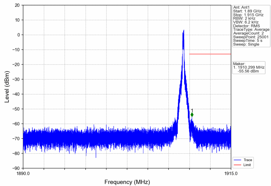
n2_15kHz_SISO_NTNV_20MHz_CP-OFDM QPSK_1900MHz_Inner_1RB_Right
