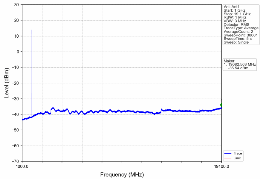
n2_15kHz_SISO_NTNV_20MHz_CP-OFDM_QPSK_1880MHz_Edge_1RB_Left
