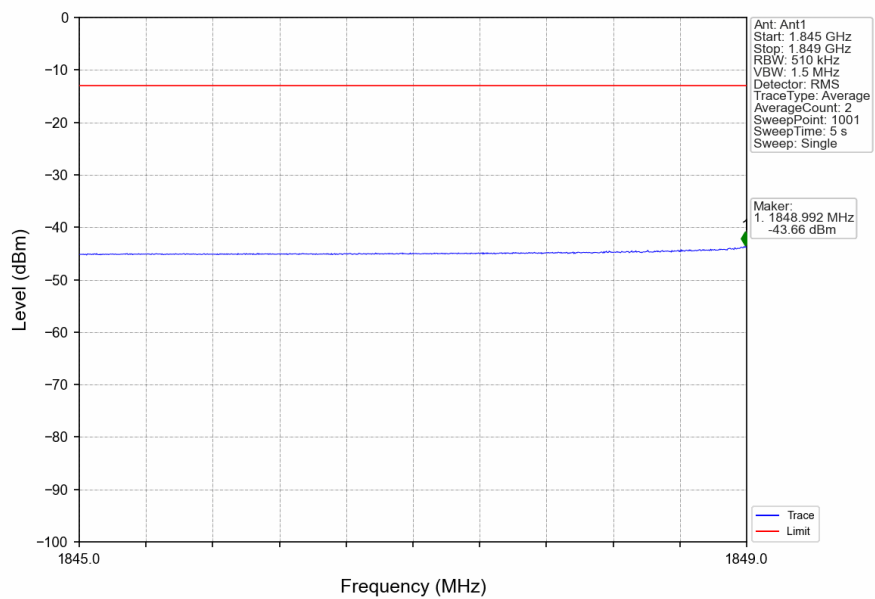
n2_15kHz_SISO_NTNV_20MHz_CP-OFDM_QPSK_1860MHz_Inner_1RB_Left
