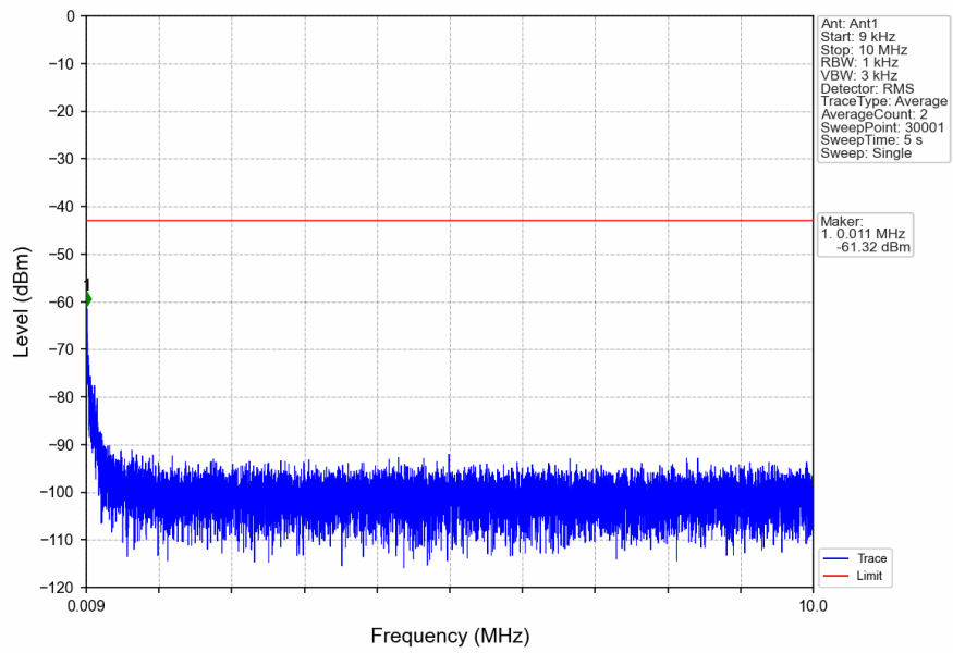
n2_15kHz_SISO_NTNV_20MHz_CP-OFDM_QPSK_1880MHz_Edge_1RB_Left
