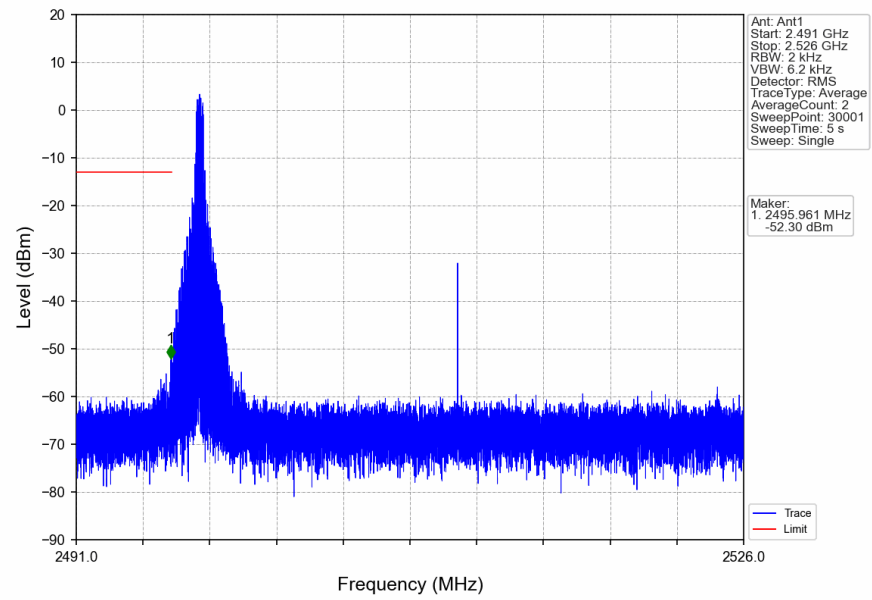
n41_30kHz_SISO_NTNV_30MHz_DFT-s-OFDM_QPSK_2511MHz_Inner_1RB_Left
