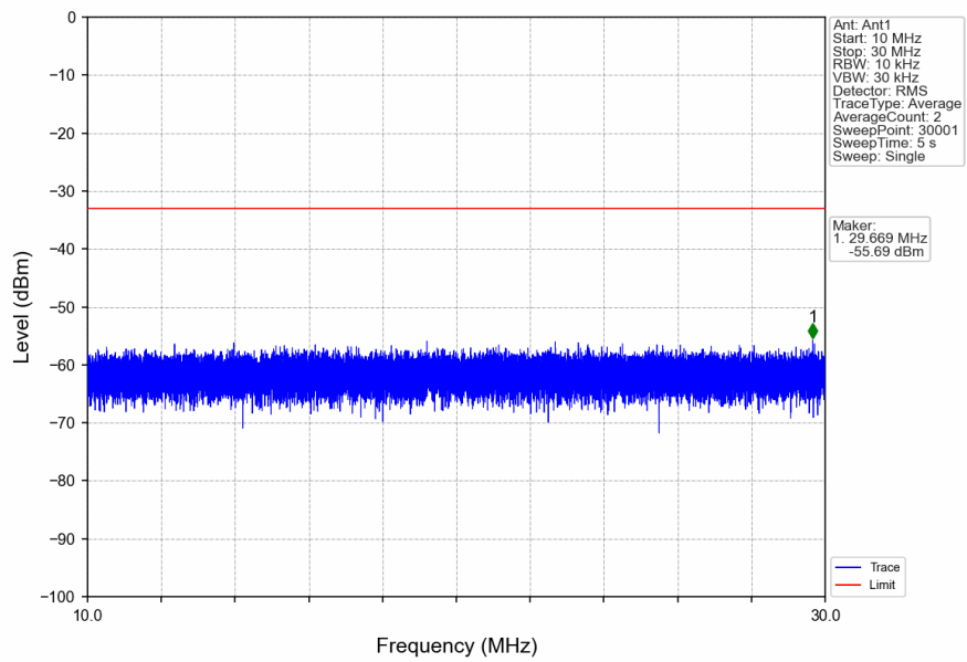
n41_30kHz_SISO_NTNV_30MHz_DFT-s-OFDM_QPSK_2511MHz_Inner_1RB_Left
