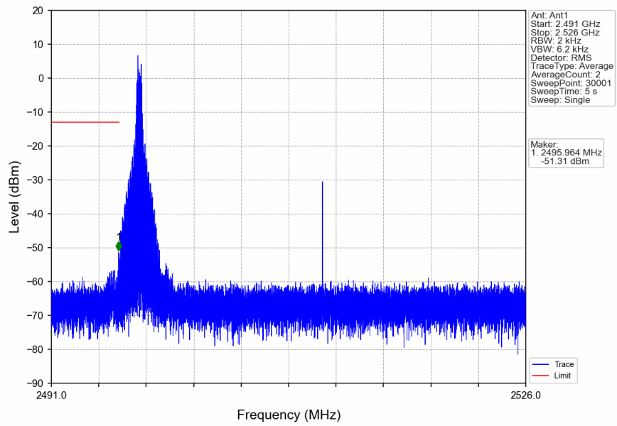
n41_30kHz_SISO_NTNV_30MHz_CP-OFDM_QPSK_2511MHz_Inner_1RB_Left
