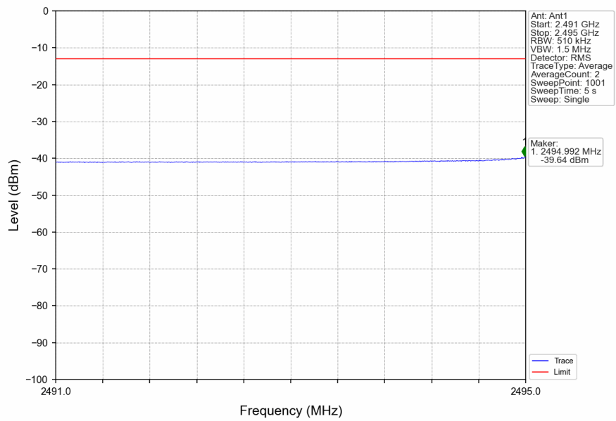
n41_30kHz_SISO_NTNV_30MHz_CP-OFDM_QPSK_2511MHz_Inner_1RB_Left
