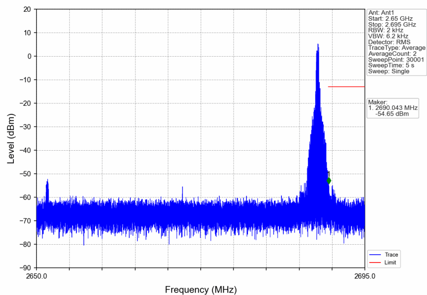
n41_30kHz_SISO_NTNV_40MHz_DFT-s-OFDM_QPSK_2670MHz_Inner_1RB_Right
