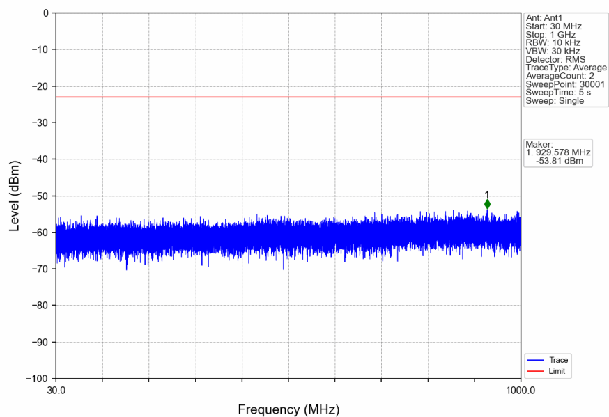
n41_30kHz_SISO_NTNV_40MHz_DFT-s-OFDM_QPSK_2670MHz_Inner_1RB_Right
