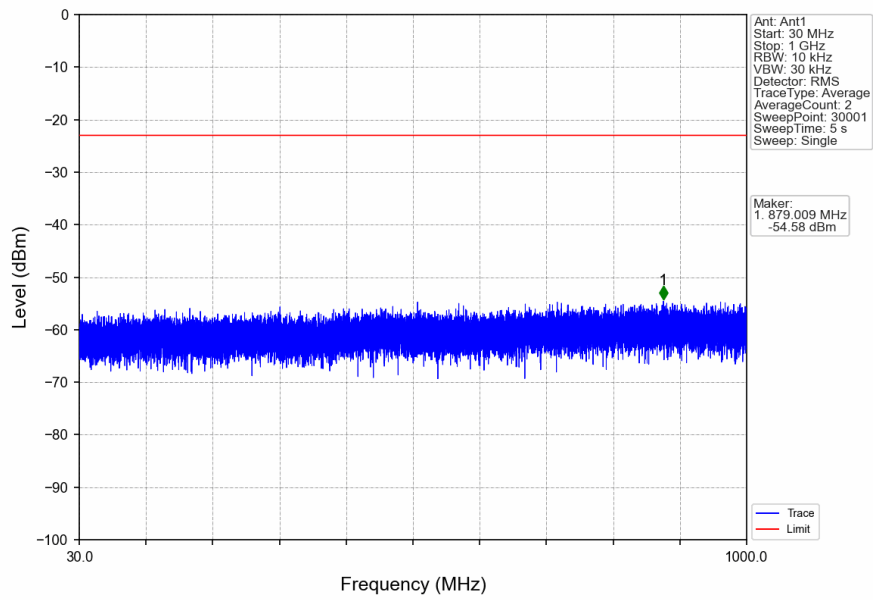
n41_30kHz_SISO_NTNV_40MHz_DFT-s-OFDM_QPSK_2516.01MHz_Inner_1RB_Left
