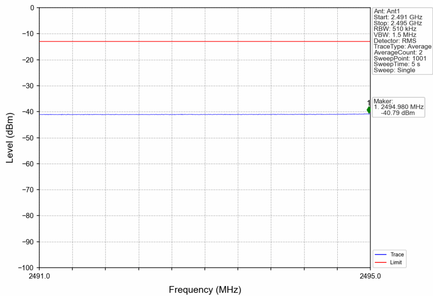
n41_30kHz_SISO_NTNV_40MHz_DFT-s-OFDM_QPSK_2516.01MHz_Inner_1RB_Left
