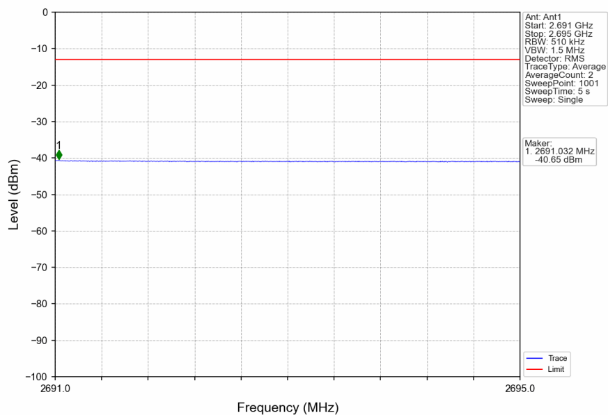
n41_30kHz_SISO_NTNV_40MHz_DFT-s-OFDM_QPSK_2670MHz_Inner_1RB_Right
