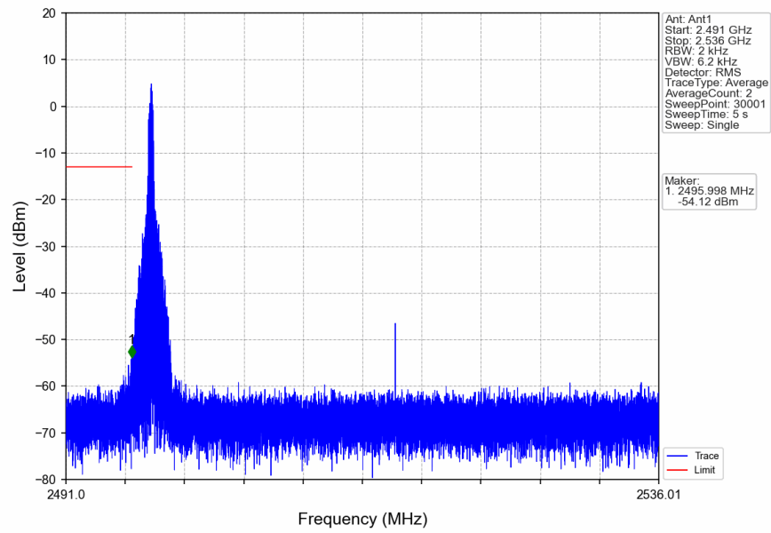
n41_30kHz_SISO_NTNV_40MHz_DFT-s-OFDM_QPSK_2516.01MHz_Inner_1RB_Left
