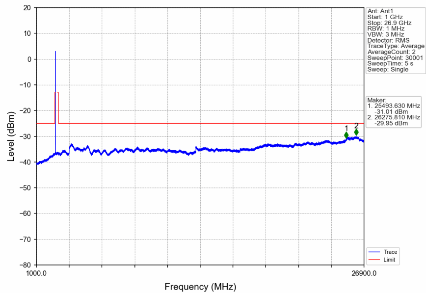
n41_30kHz_SISO_NTNV_40MHz_DFT-s-OFDM_QPSK_2516.01MHz_Inner_1RB_Left
