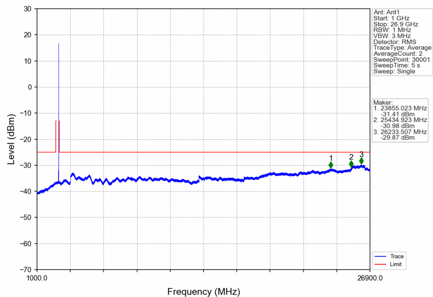
n41_30kHz_SISO_NTNV_40MHz_DFT-s-OFDM_QPSK_2670MHz_Inner_1RB_Right
