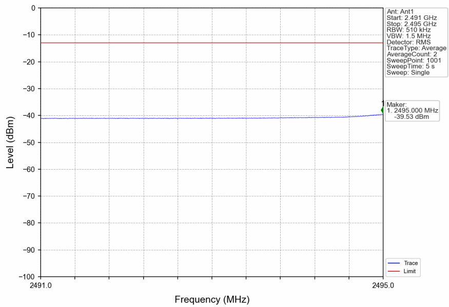
n41_30kHz_SISO_NTNV_60MHz_DFT-s-OFDM_PI/2_BPSK_2526MHz_Inner_1RB_Left
