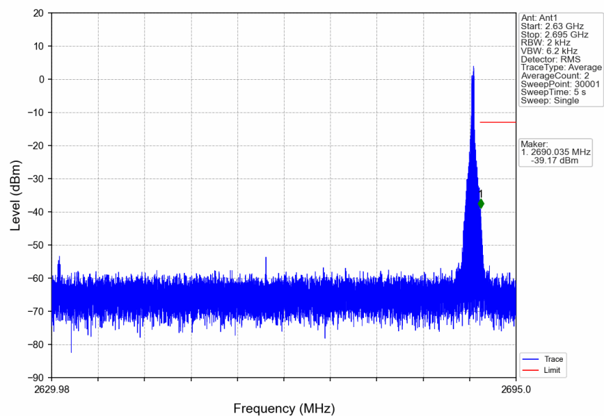
n41_30kHz_SISO_NTNV_60MHz_DFT-s-OFDM_PI/2_BPSK_2659.98MHz_Edge_1RB_Right
