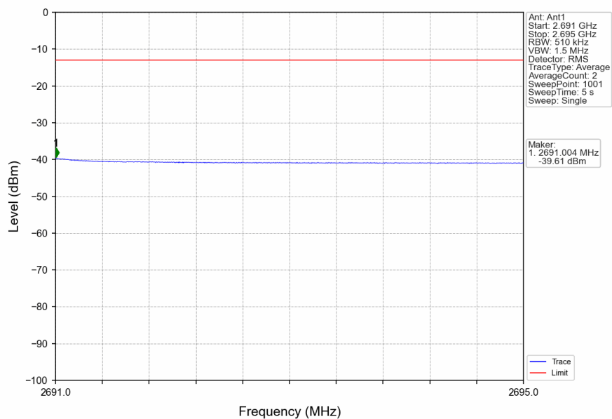
n41_30kHz_SISO_NTNV_60MHz_DFT-s-OFDM_PI/2_BPSK_2659.98MHz_Inner_1RB_Right
