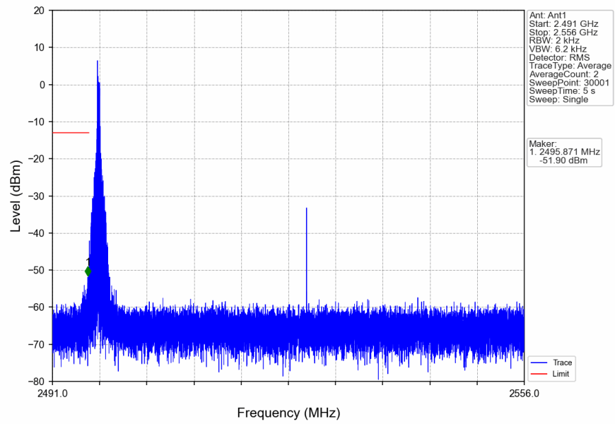
n41_30kHz_SISO_NTNV_60MHz_DFT-s-OFDM_PI/2_BPSK_2526MHz_Inner_1RB_Left
