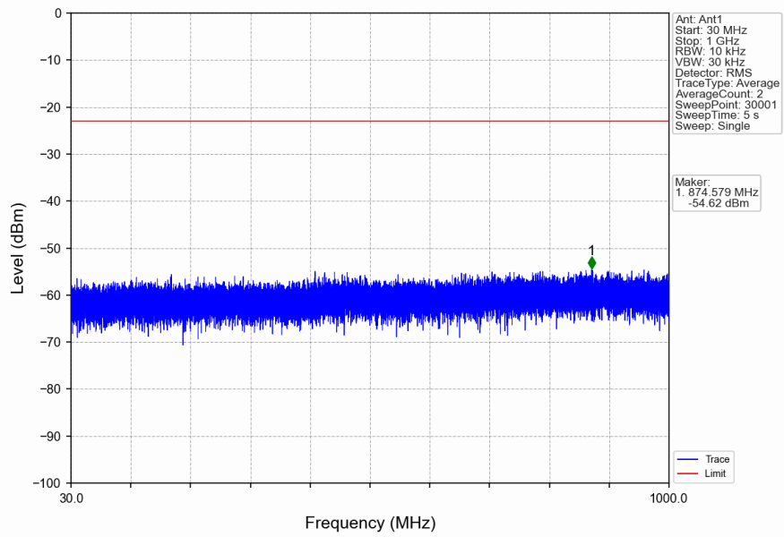
n41_30kHz_SISO_NTNV_50MHz_CP-OFDM_QPSK_2521.02MHz_Inner_1RB_Left
