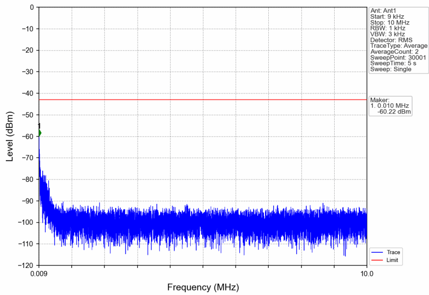
n41_30kHz_SISO_NTNV_60MHz_DFT-s-OFDM_QPSK_2526MHz_Edge_1RB_Left
