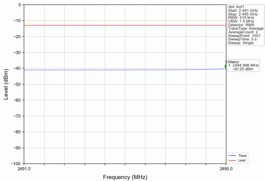
n41_30kHz_SISO_NTNV_50MHz_CP-OFDM_QPSK_2521.02MHz_Inner_1RB_Left
