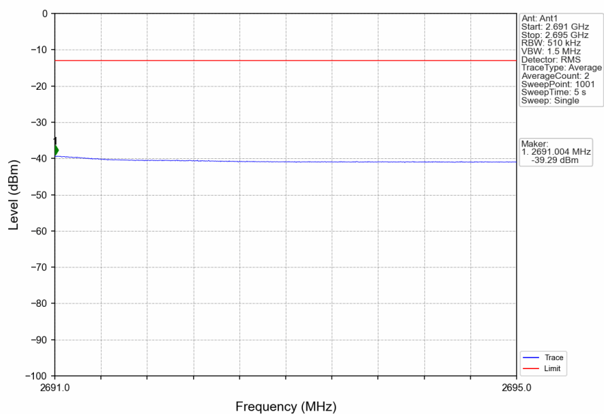
n41_30kHz_SISO_NTNV_60MHz_DFT-s-OFDM_PI/2_BPSK_2659.98MHz_Edge_1RB_Right
