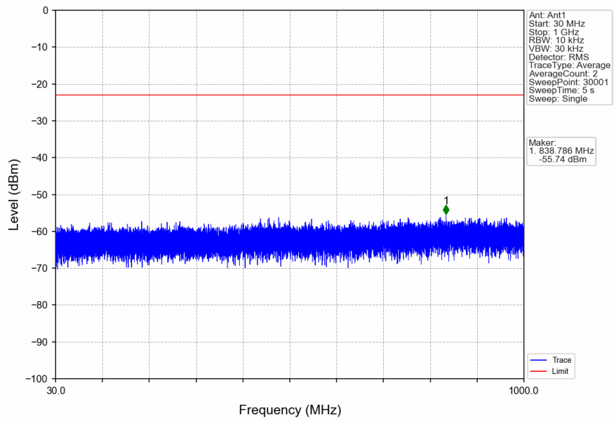
n41_30kHz_SISO_NTNV_60MHz_DFT-s-OFDM_QPSK_2526MHz_Edge_1RB_Left
