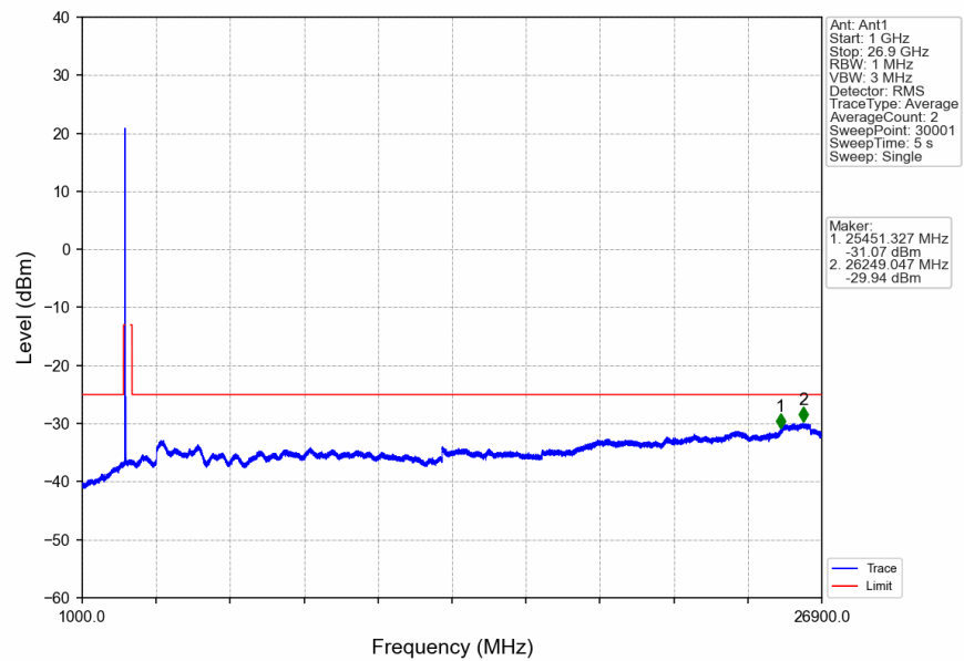
n41_30kHz_SISO_NTNV_50MHz_CP-OFDM_QPSK_2521.02MHz_Inner_1RB_Left
