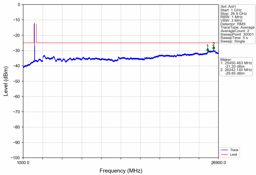
n41_30kHz_SISO_NTNV_60MHz_DFT-s-OFDM_QPSK_2526MHz_Inner_1RB_Left
