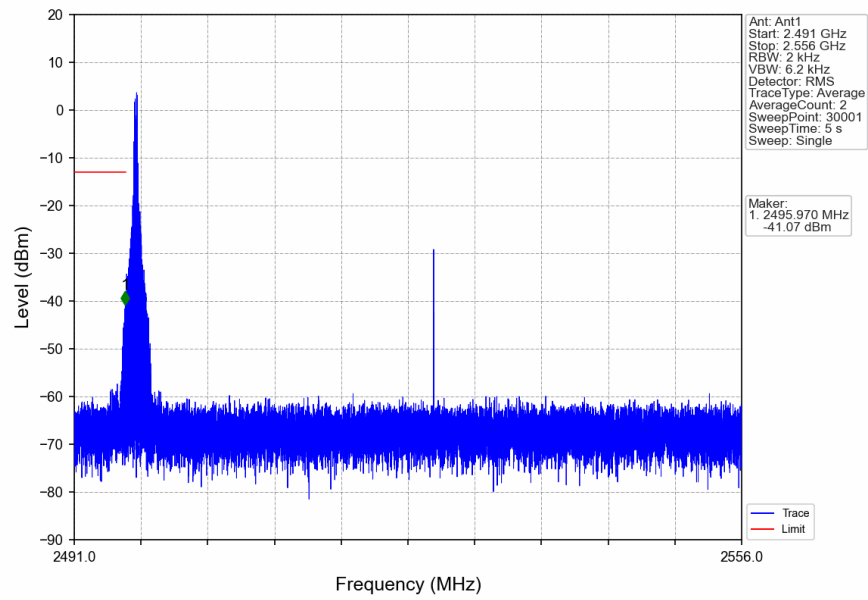
n41_30kHz_SISO_NTNV_60MHz_DFT-s-OFDM_QPSK_2526MHz_Edge_1RB_Left
