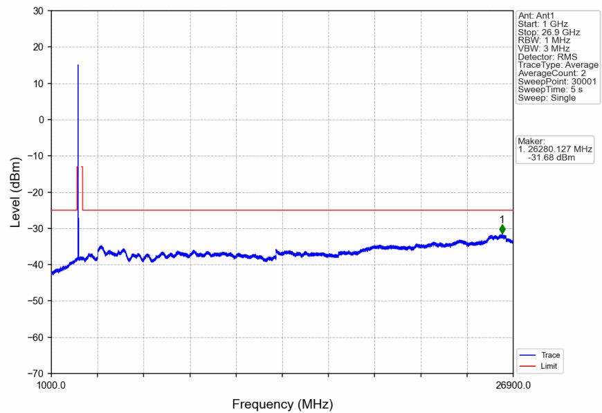
n41_30kHz_SISO_NTNV_60MHz_DFT-s-OFDM_QPSK_2526MHz_Edge_1RB_Left
