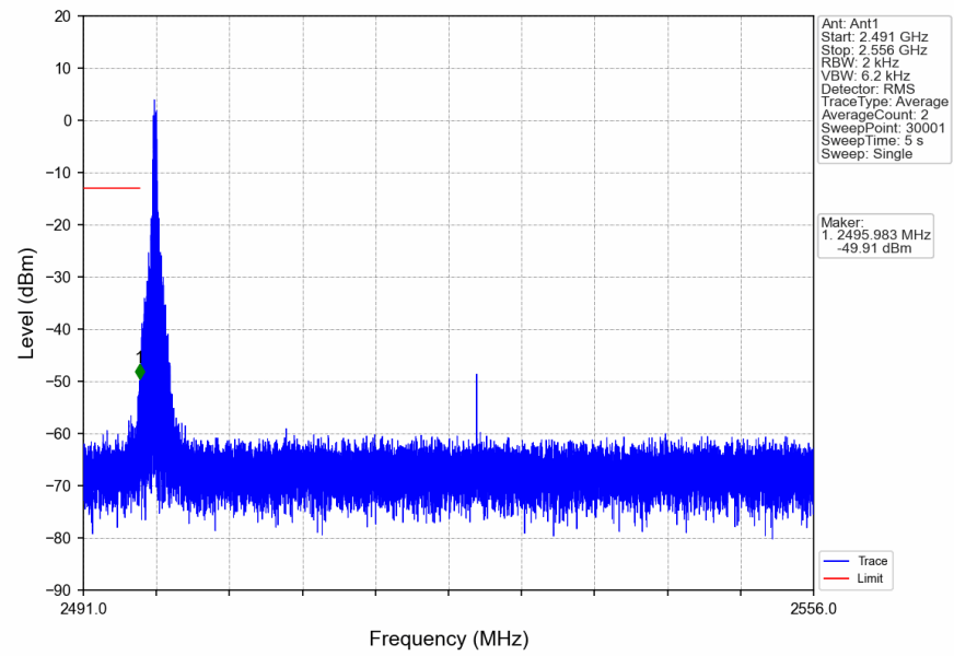
n41_30kHz_SISO_NTNV_60MHz_DFT-s-OFDM_QPSK_2526MHz_Inner_1RB_Left
