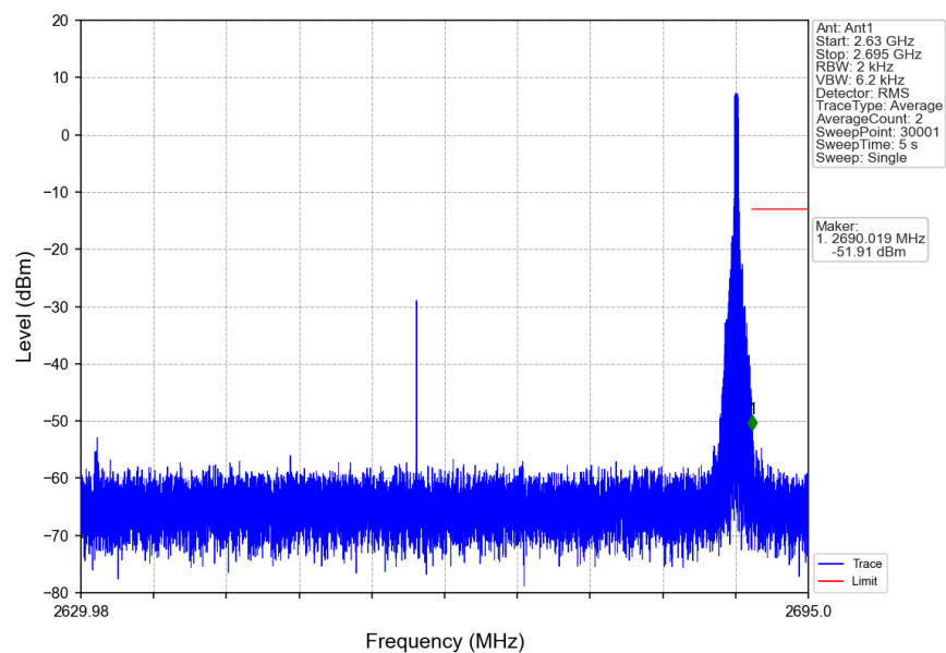
n41_30kHz_SISO_NTNV_60MHz_DFT-s-OFDM_PI/2_BPSK_2659.98MHz_Inner_1RB_Right
