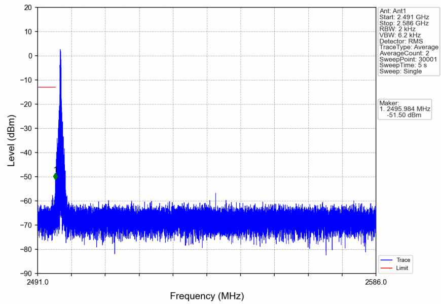
n41_30kHz_SISO_NTNV_90MHz_DFT-s-OFDM_PI/2_BPSK_2541MHz_Inner_1RB_Left
