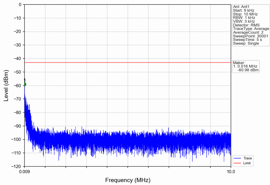
n41_30kHz_SISO_NTNV_80MHz_CP-OFDM_QPSK_2536.02MHz_Inner_1RB_Left
