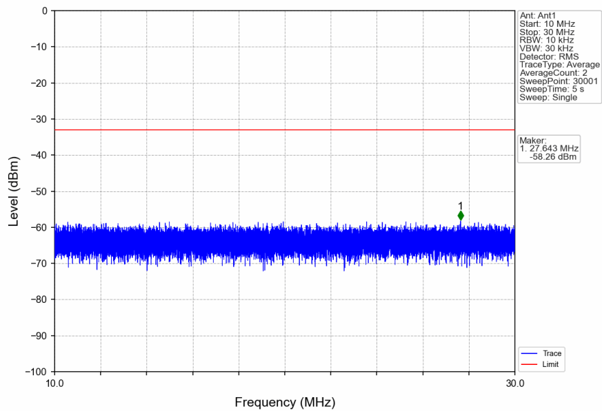
n41_30kHz_SISO_NTNV_80MHz_CP-OFDM_QPSK_2536.02MHz_Inner_1RB_Left
