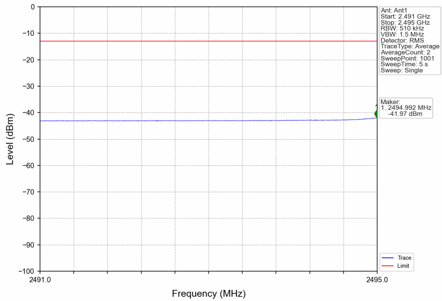
n41_30kHz_SISO_NTNV_90MHz_DFT-s-OFDM_PI/2_BPSK_2541MHz_Inner_1RB_Left
