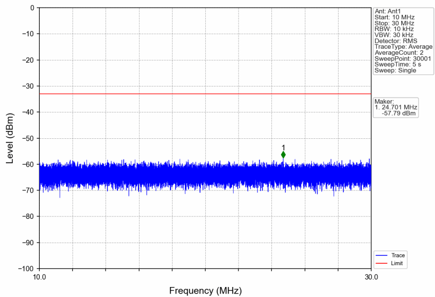
n41_30kHz_SISO_NTNV_90MHz_DFT-s-OFDM_QPSK_2541MHz_Inner_1RB_Left
