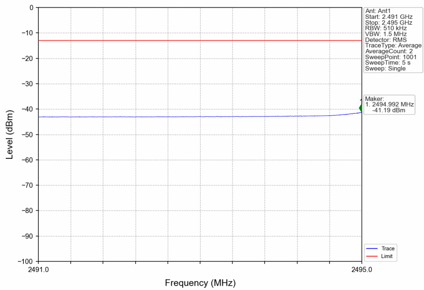
n41_30kHz_SISO_NTNV_90MHz_CP-OFDM_QPSK_2541MHz_Inner_1RB_Left
