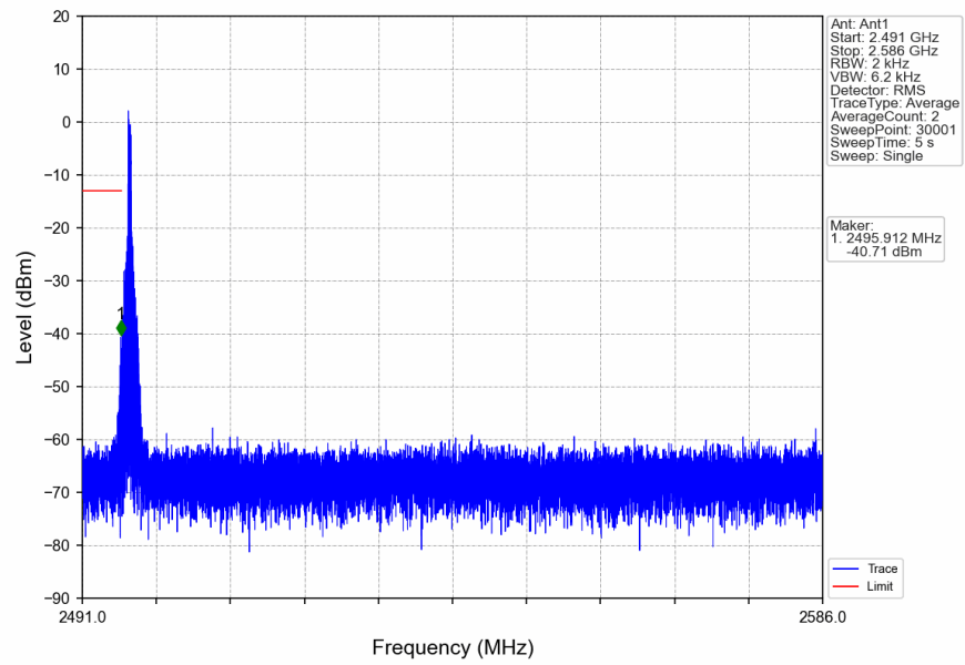
n41_30kHz_SISO_NTNV_90MHz_CP-OFDM_QPSK_2541MHz_Edge_1RB_Left
