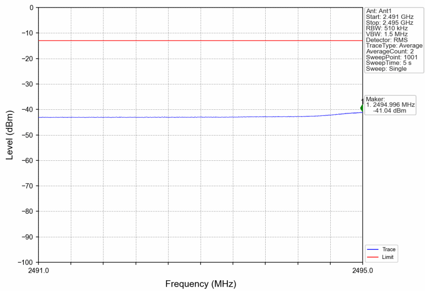
n41_30kHz_SISO_NTNV_90MHz_CP-OFDM_QPSK_2541MHz_Edge_1RB_Left
