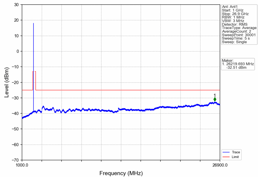
n41_30kHz_SISO_NTNV_90MHz_DFT-s-OFDM_QPSK_2541MHz_Inner_1RB_Left
