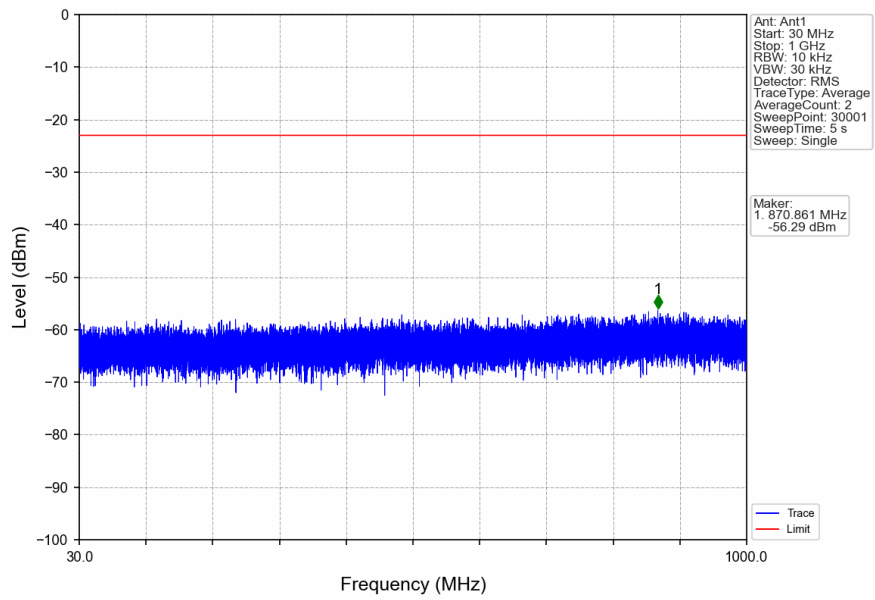
n41_30kHz_SISO_NTNV_90MHz_DFT-s-OFDM_QPSK_2541MHz_Inner_1RB_Left
