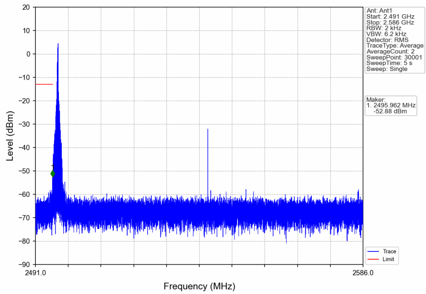
n41_30kHz_SISO_NTNV_90MHz_CP-OFDM_QPSK_2541MHz_Inner_1RB_Left
