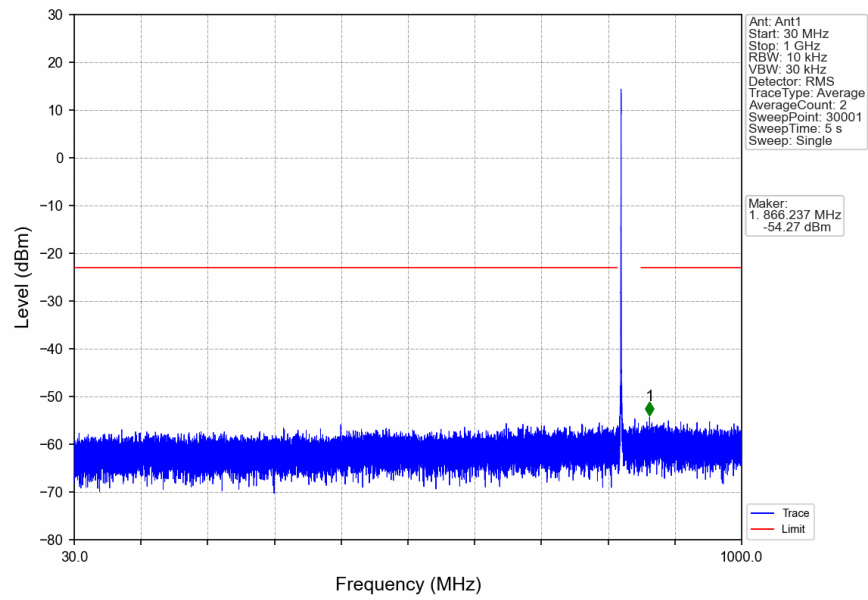
n5_15kHz_SISO_NTNV_20MHz_DFT-s-OFDM PI/2 BPSK_834MHz_Inner_1RB_Left
