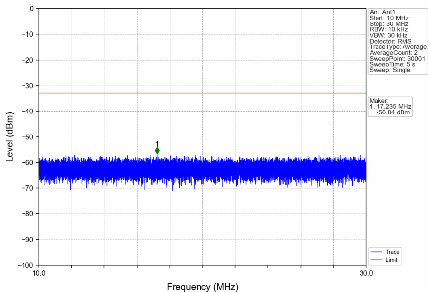
n5_15kHz_SISO_NTNV_20MHz_DFT-s-OFDM PI/2 BPSK_834MHz_Inner_1RB_Left
