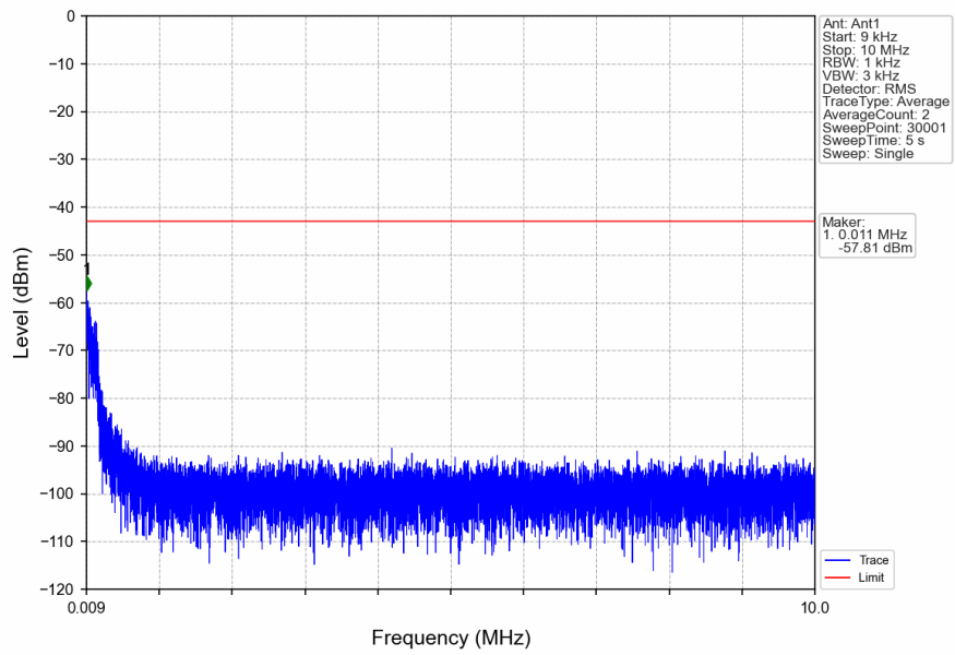
n5_15kHz_SISO_NTNV_20MHz_CP-OFDM_QPSK_834MHz_Inner_1RB_Left
