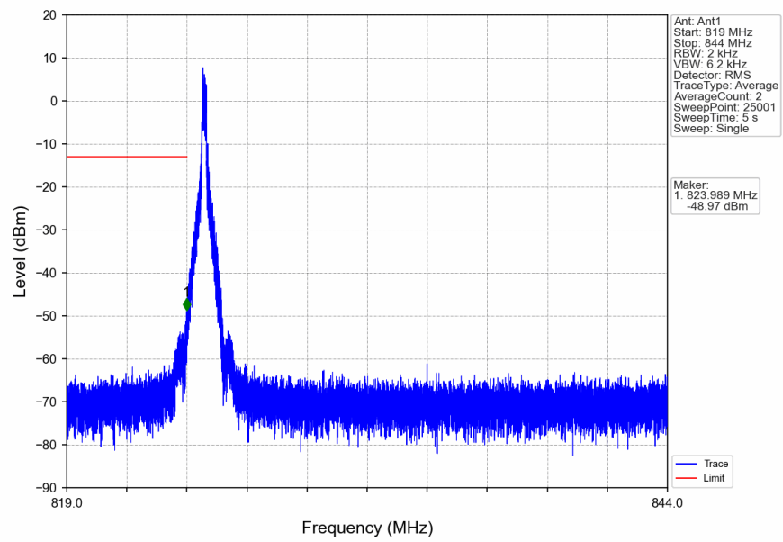
n5_15kHz_SISO_NTNV_20MHz_CP-OFDM_QPSK_834MHz_Inner_1RB_Left
