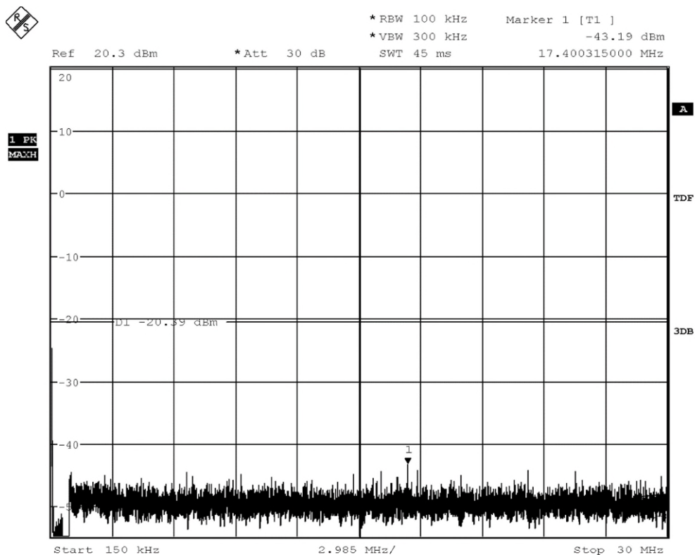
20dBc_0.15MHz-30MHz_REF_2412_2Mbit
