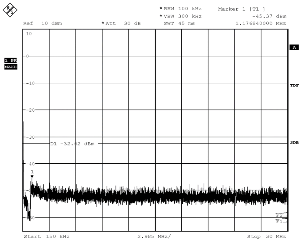
20dBc_0.15MHz-30MHz_2422_nmode_HT40_MCS0
