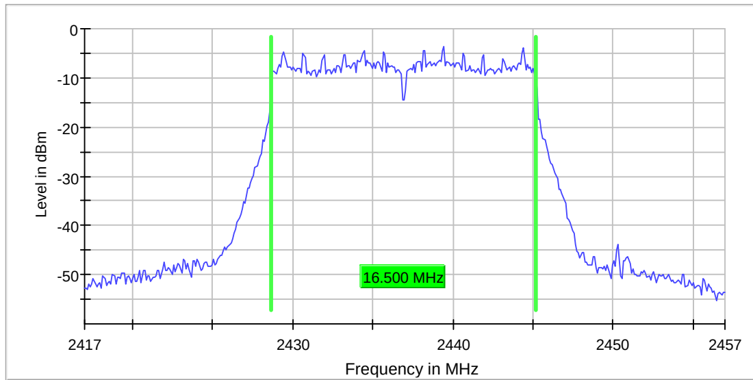
6dB_BW_CH06_g-mode_6MBIT
