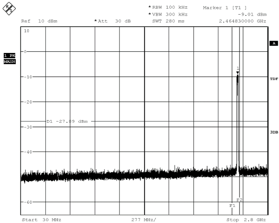
20dBc_0.30MHz-2.8Ghz_2462_nmode_MCS3
