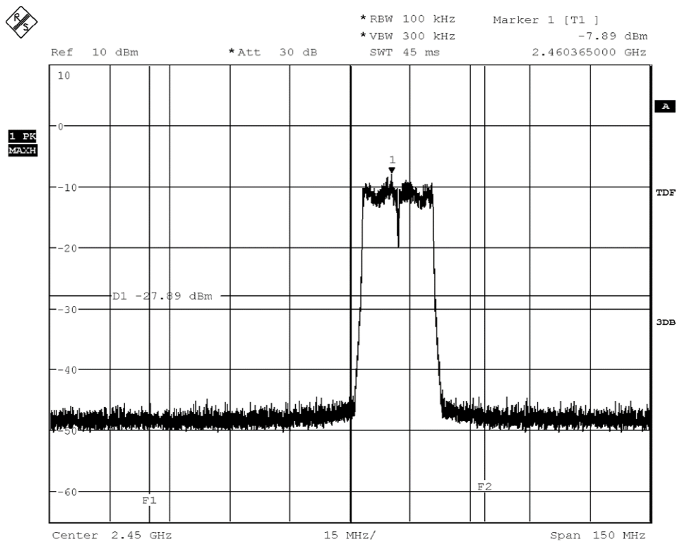
20dBc_REF_2462_nmode_MCS3
