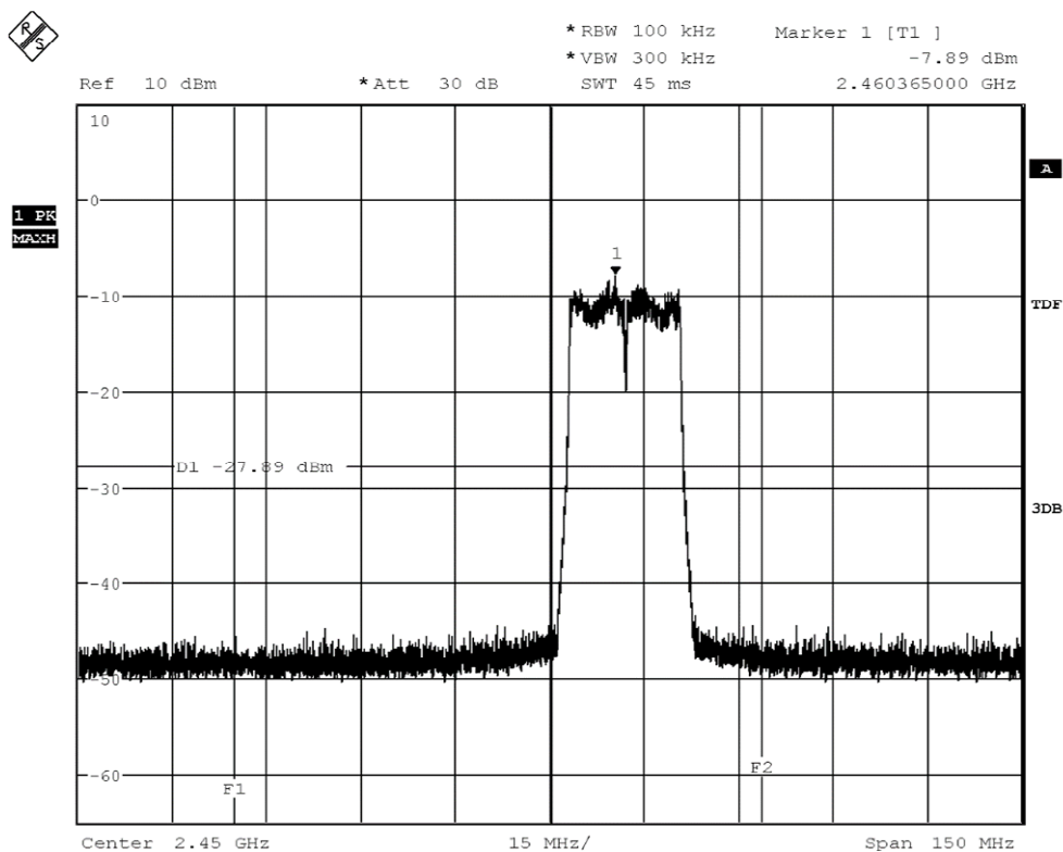
20dBc_REF_2462_nmode_MCS3
