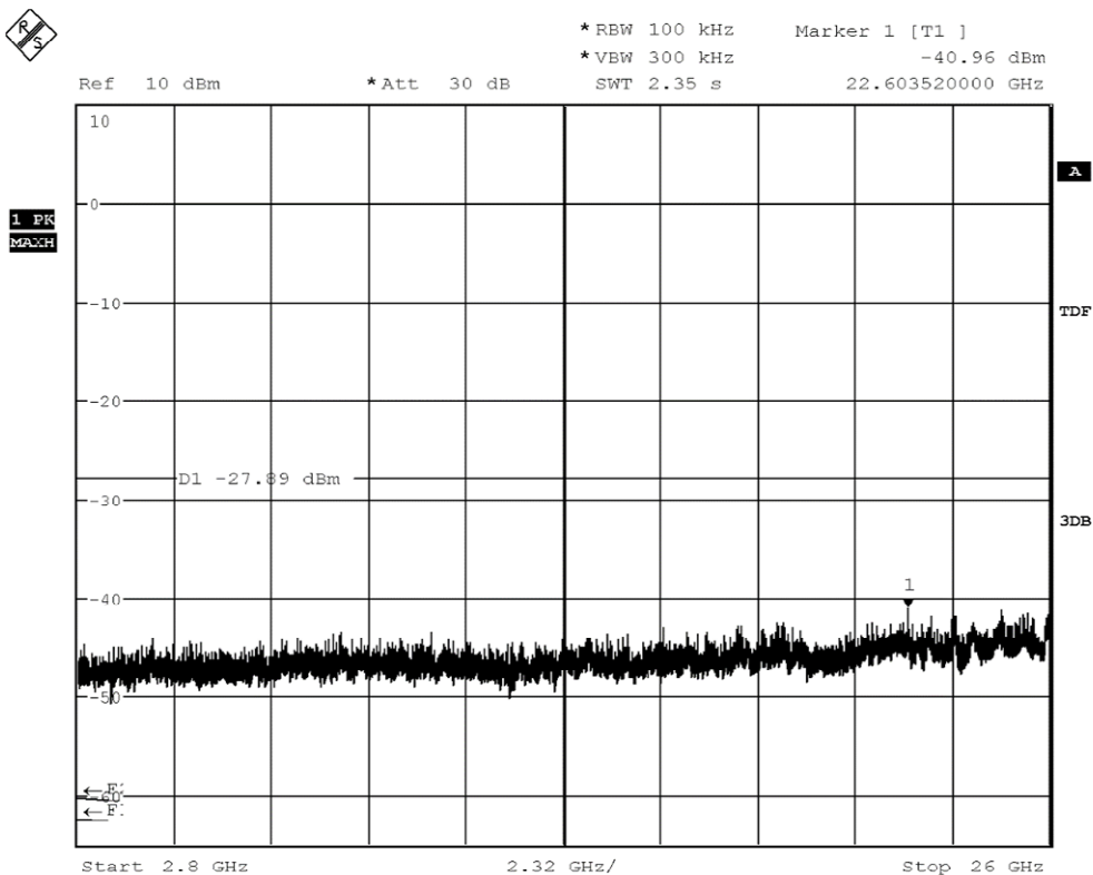
20dBc_2.8GHz-26Ghz_2462_nmode_MCS3
