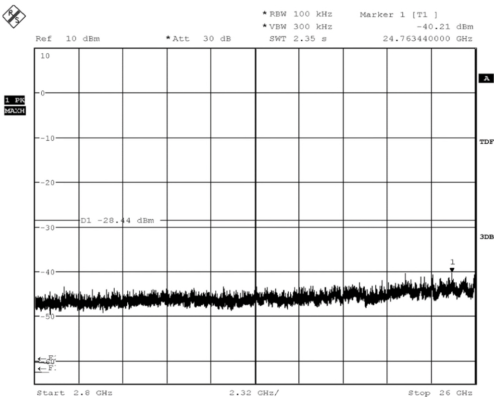
20dBc_2.8GHz-26Ghz_gmode_6Mbit
