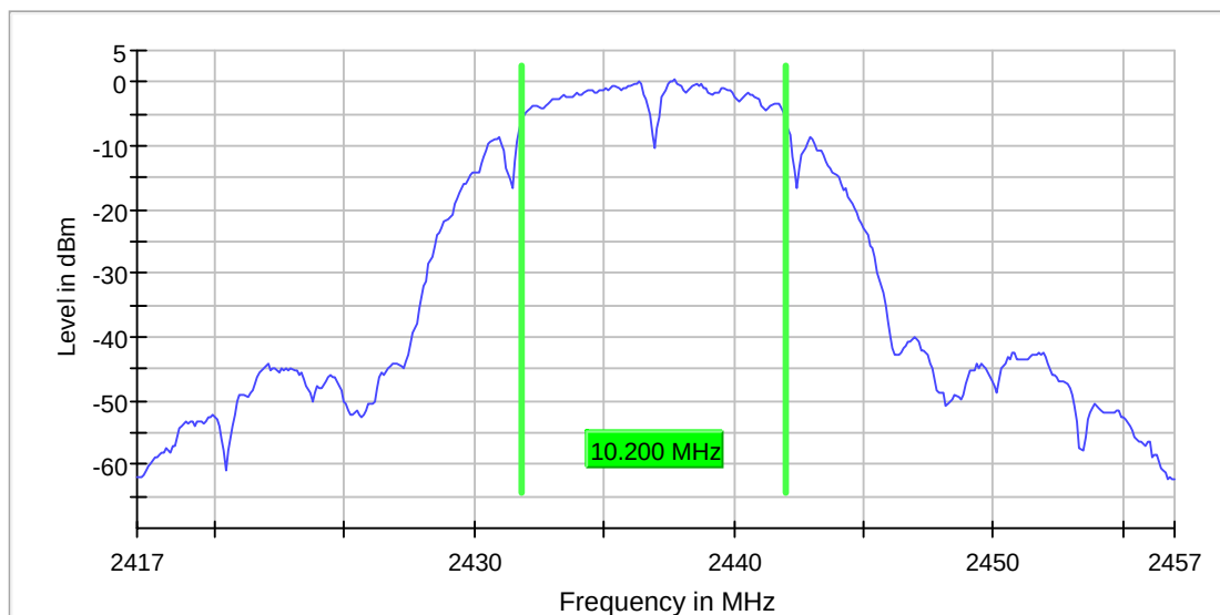
6dB_BW_CH06_bmode_2MBIT
