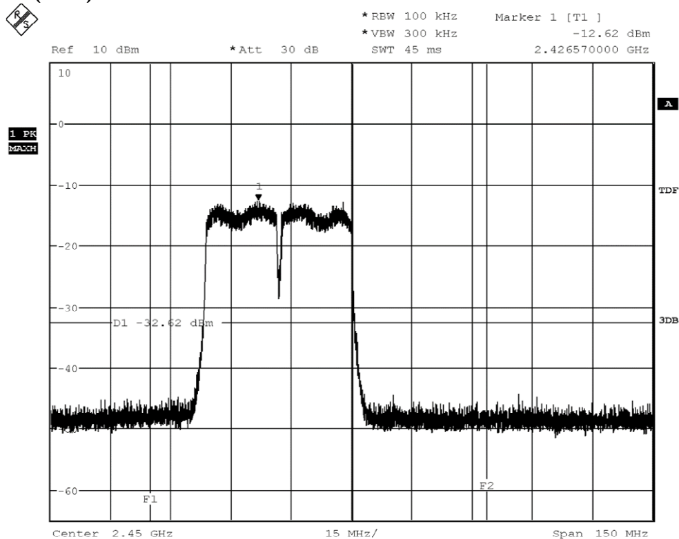
20dBc_REF_2422_nmode_HT40_MCS0
