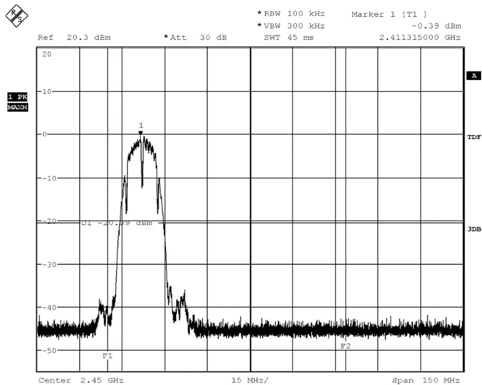
20dBc_REF_2412_bmode_2Mbit
