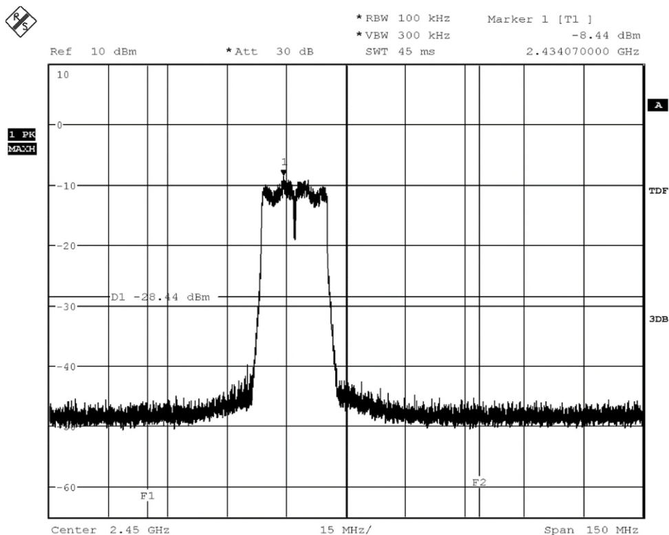
20dBc_REF_2437_gmode_6Mbit
