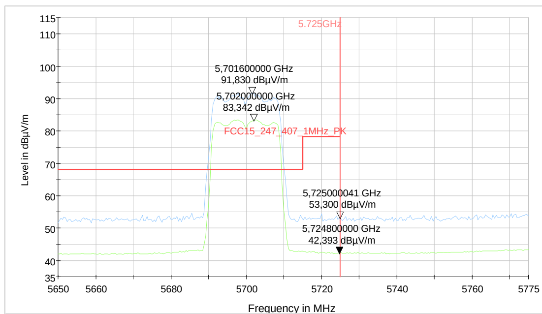
9.11b_ac-mode_MCS4_ch140
