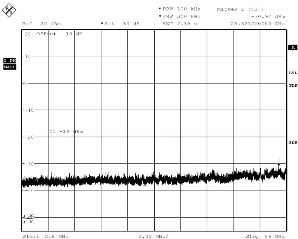
20dBc_2.8GHz-26GHz_2402_3-DH5
