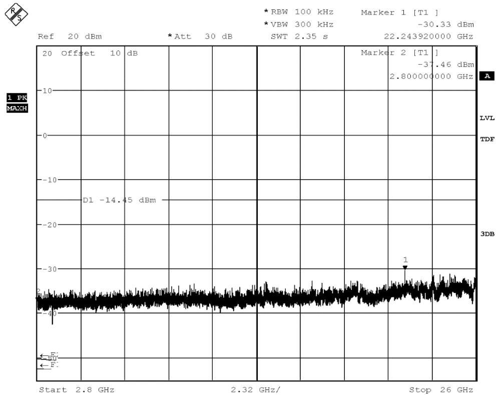
20dBc_2.8GHz-26Ghz_2441_DH5
