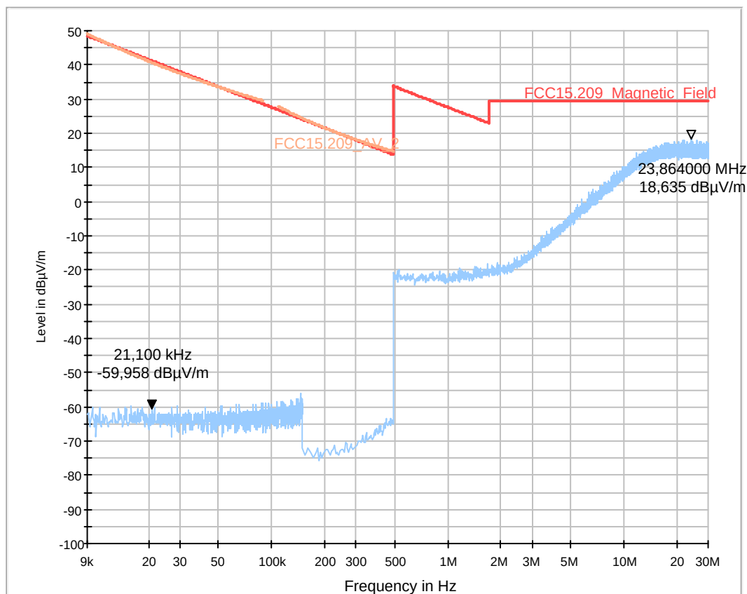
FCC15.209_magn hor+vert
