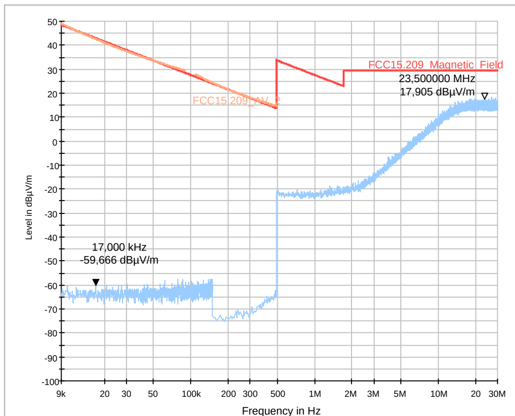
FCC15.209_magn hor+vert
