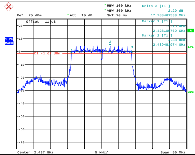
11n HT 20 CH6
