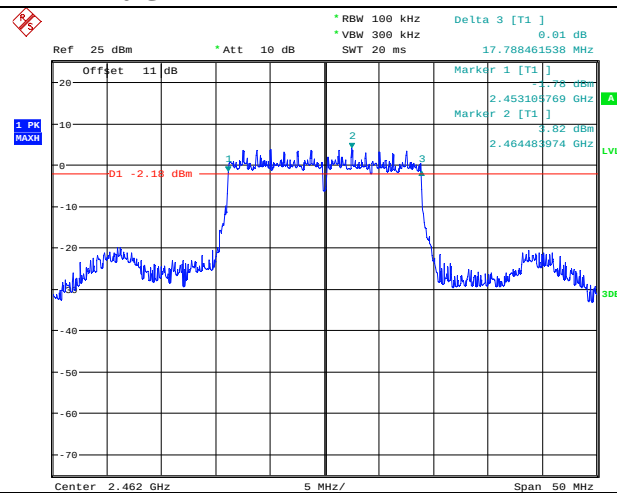
11n HT 20 CH11
