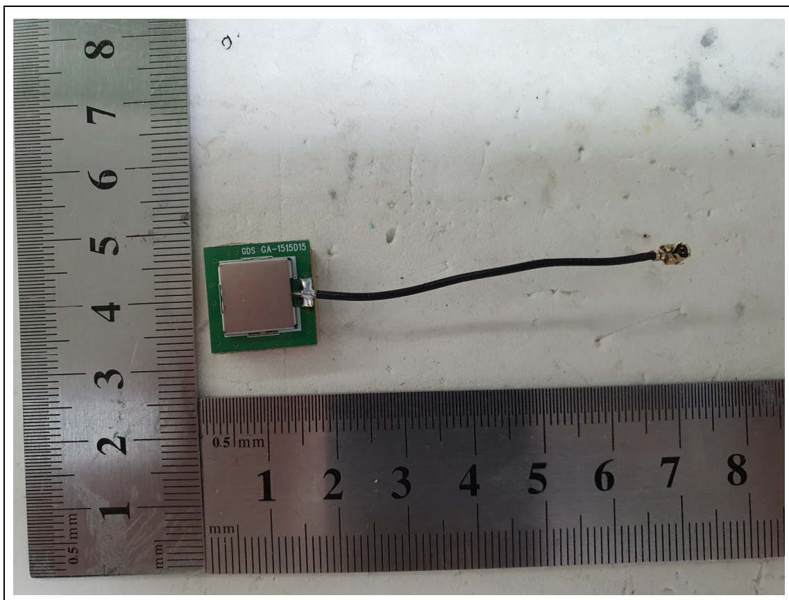
<GPS Antenna>
