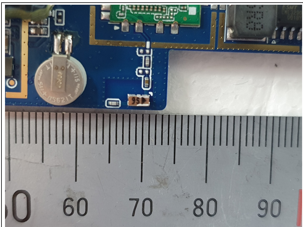
<WLAN/BT Antenna>
