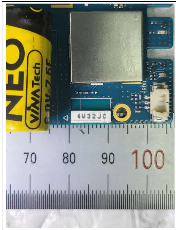
<WLAN Antenna>
