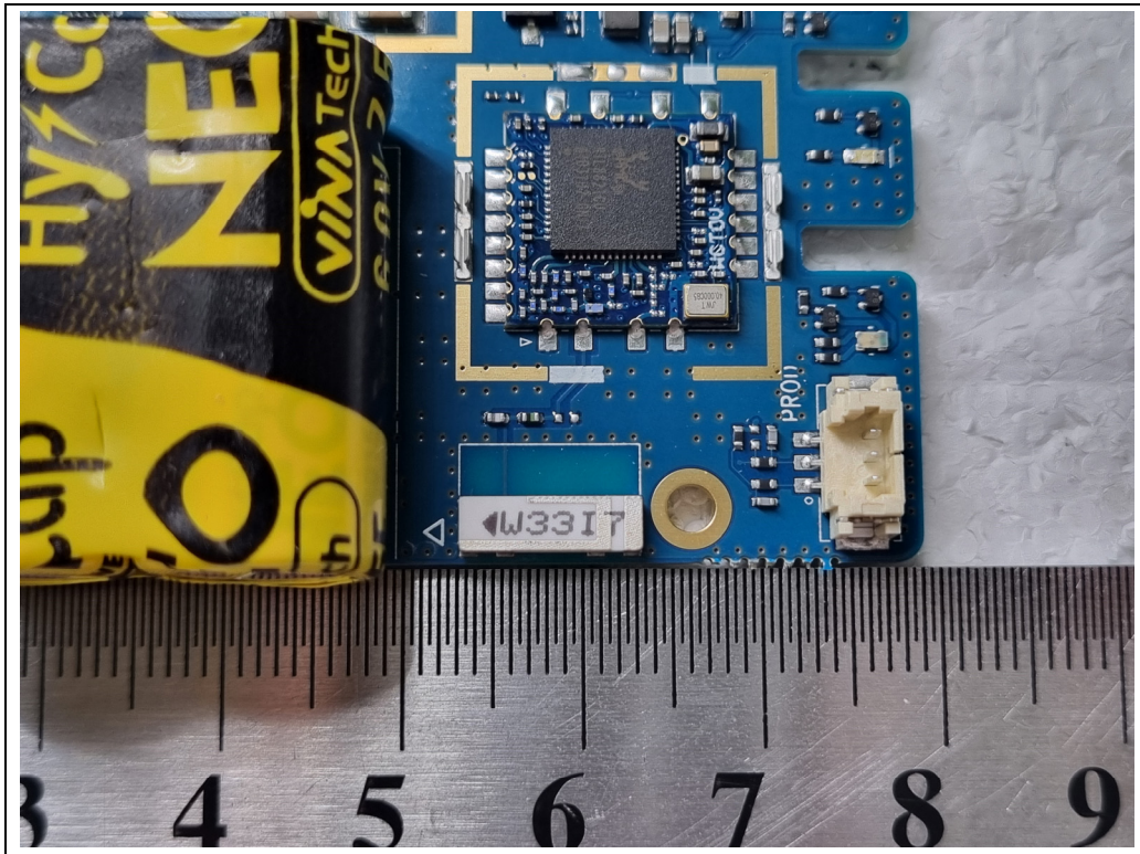
<WLAN Module & Antenna>
