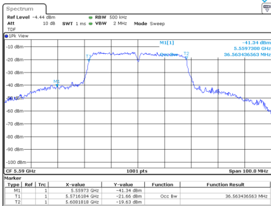
UNII-2C / 802.11n(HT40)/ 5 590 MHz
