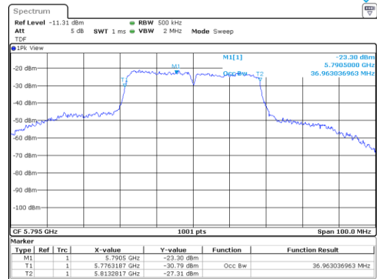
UNII-3 / 802.ac(VHT40)/ 5 795 MHz
