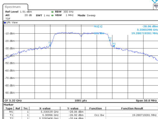
UNII-2A / 802.11ac(VHT20)/ 5 320 MHz
