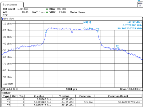
UNII-2C / 802.ac(VHT40)/ 5 670 MHz
