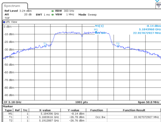
UNII-1 / 802.11ac(VHT20) / 5 180 MHz
