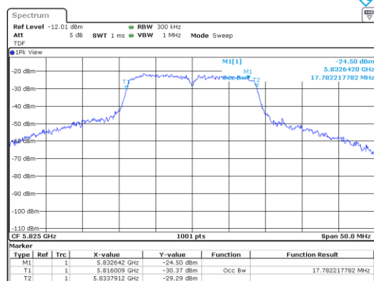
UNII-3 / 802.11n(HT20)/ 5 825 MHz
