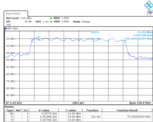
UNII-2A / 802.ac(VHT80)/ 5 290 MHz
