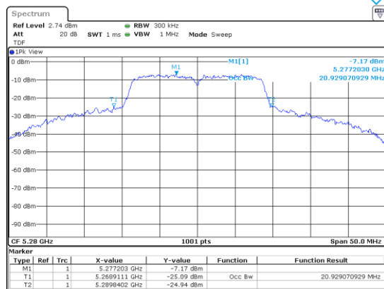
UNII-2A / 802.11ac(VHT20)/ 5 280 MHz
