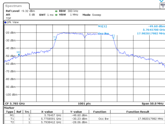
UNII-3 / 802.11n(HT20)/ 5 785 MHz
