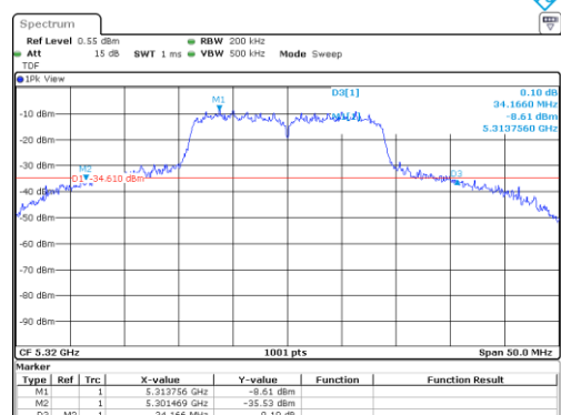
UNII-2A / 802.11n(HT20)/ 5 320 MHz
