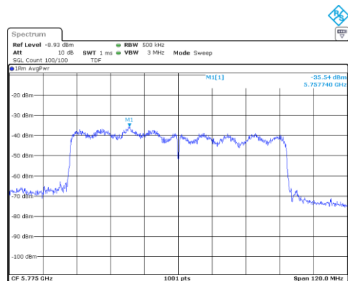
UNII-3 / 802.11ac(VHT80)/ 5 775 MHz
