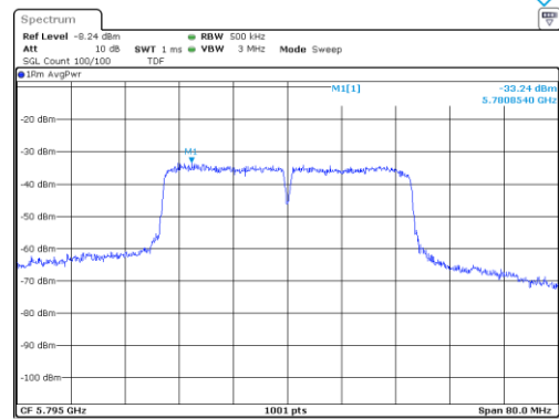
UNII-3 / 802.11ac(VHT40)/ 5 795 MHz
