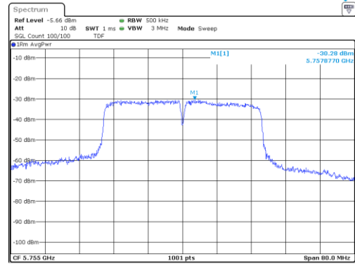
UNII-3 / 802.11ac(VHT40)/ 5 755 MHz
