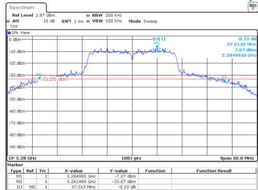
UNII-2A / 802.11n(HT20)/ 5 280 MHz
