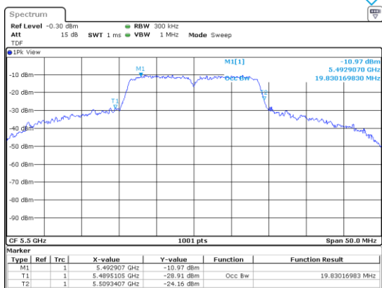
UNII-2C / 802.11n(HT20)/ 5 500 MHz
