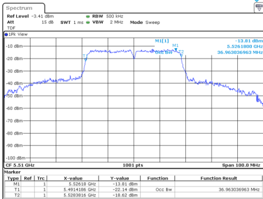
UNII-2C / 802.11n(HT40)/ 5 510 MHz
