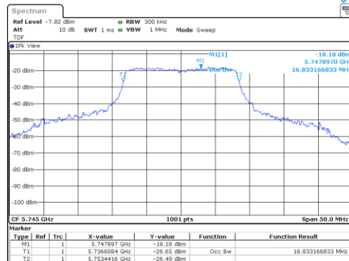
UNII-3 / 802.11a / 5 745 MHz
