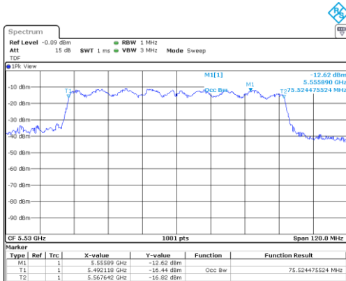
UNII-2C / 802.ac(VHT80)/ 5 530 MHz
