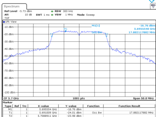
UNII-2C / 802.11n(HT20)/ 5 700 MHz
