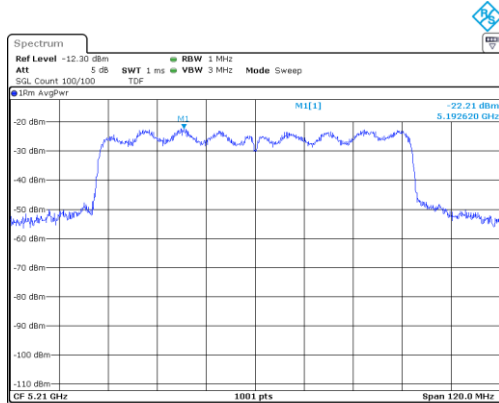
UNII-1 / 802.11ac(VHT80)/ 5 210 MHz
