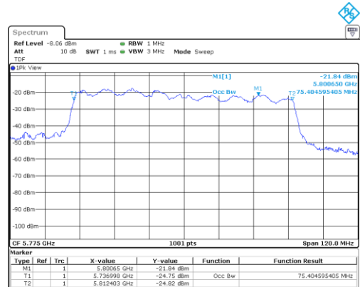
UNII-3 / 802.ac(VHT80)/ 5 775 MHz
