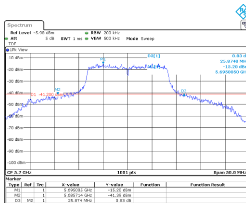
UNII-2C / 802.11a / 5 700 MHz
