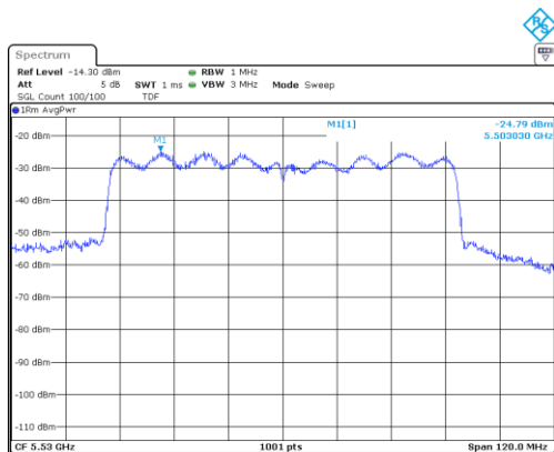
UNII-2C / 802.11ac(VHT80)/ 5 530 MHz
