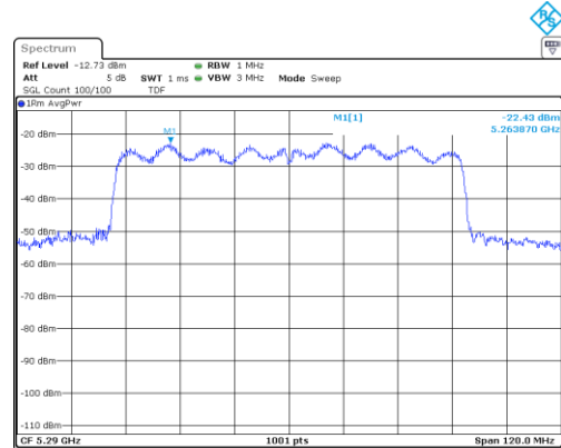
UNII-2A / 802.11ac(VHT80)/ 5 290 MHz
