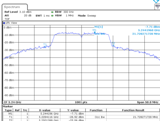
UNII-1 / 802.11ac(VHT20)/ 5 240 MHz
