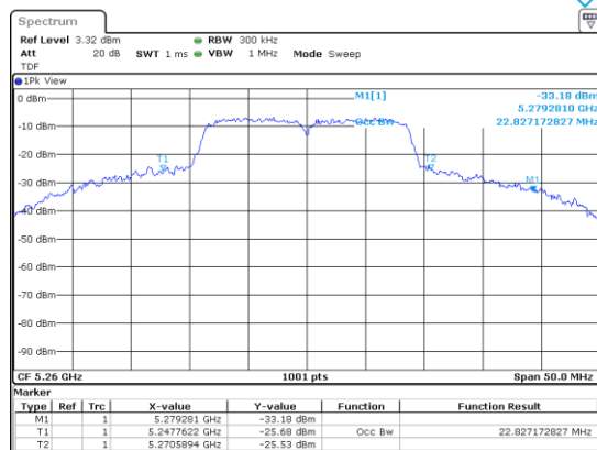
UNII-2A / 802.11ac(VHT20)/ 5 260 MHz
