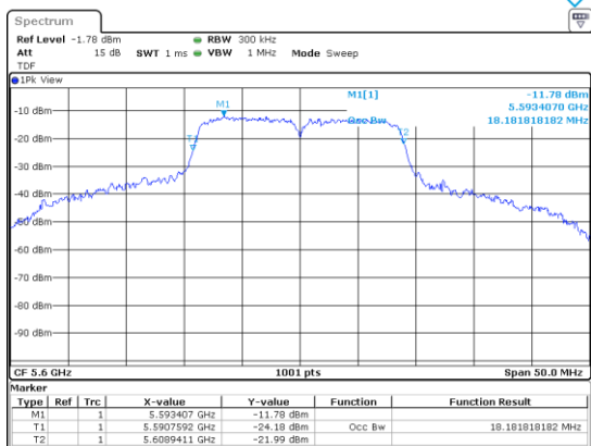
UNII-2C / 802.11n(HT20)/ 5 600 MHz
