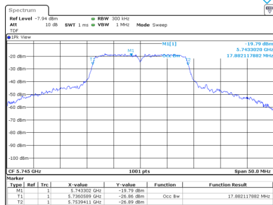
UNII-3 / 802.11n(HT20)/ 5 745 MHz
