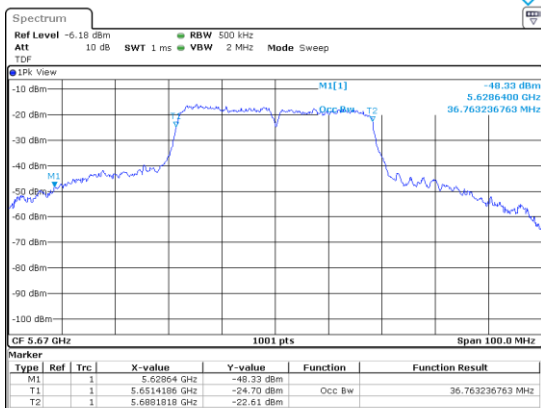
UNII-2C / 802.11n(HT40)/ 5 670 MHz
