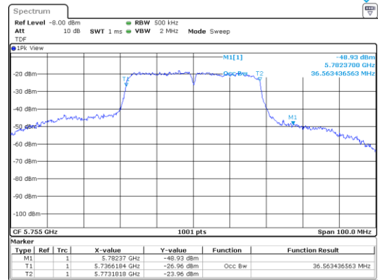
UNII-3 / 802.ac(VHT40)/ 5 755 MHz
