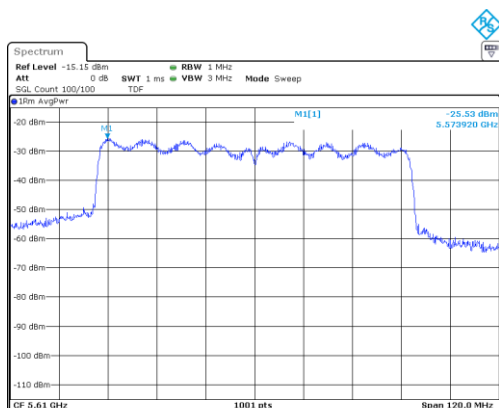
UNII-2C / 802.11ac(VHT80)/ 5 610 MHz
