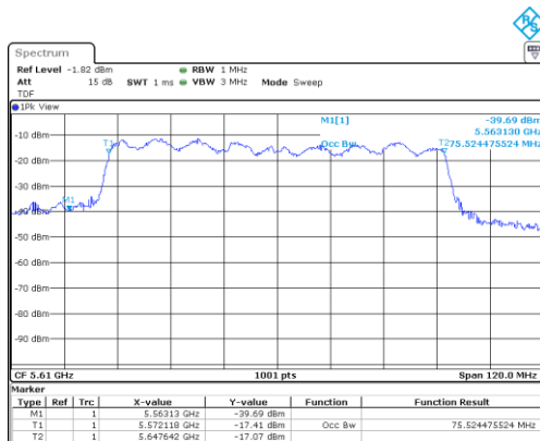
UNII-2C / 802.ac(VHT80)/ 5 610 MHz
