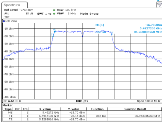
UNII-2C / 802.ac(VHT40)/ 5 510 MHz
