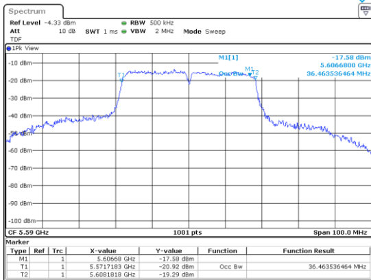
UNII-2C / 802.ac(VHT40)/ 5 590 MHz
