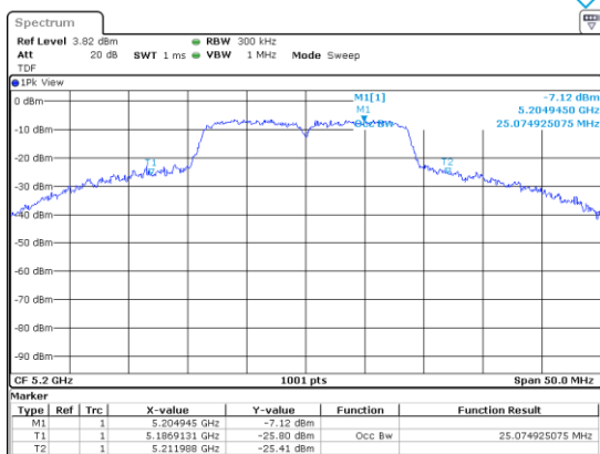
UNII-1 / 802.11ac(VHT20)/ 5 200 MHz
