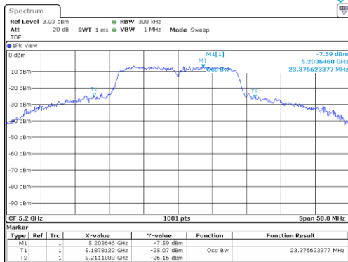
UNII-1 / 802.11n(HT20) / 5 200 MHz
