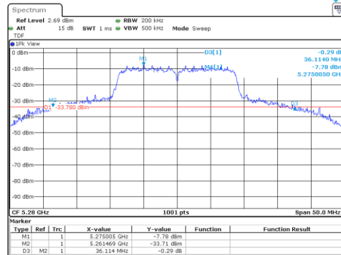
UNII-2A / 802.11n(HT20) / 5 280 MHz
