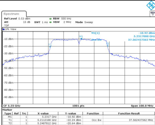
UNII-1 / 802.ac(VHT40)/ 5 230 MHz
