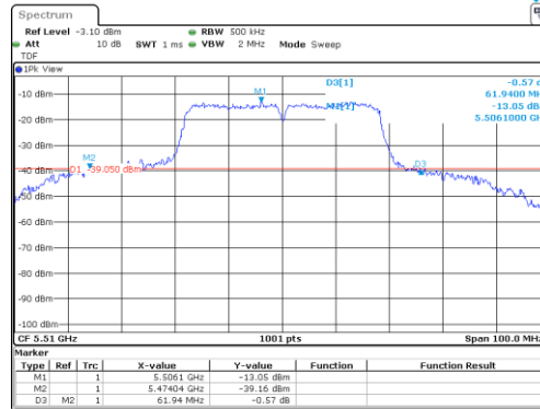
UNII-2C / 802.11ac(VHT40)/ 5 510 MHz
