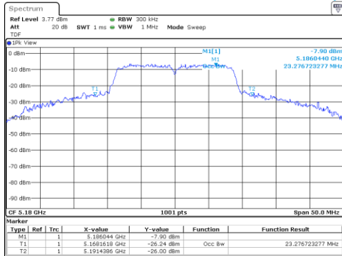
UNII-1 / 802.11n(HT20) / 5 180 MHz
