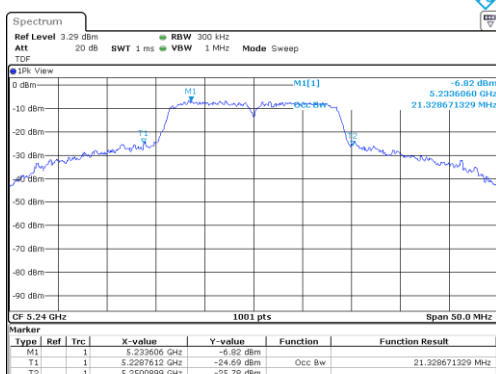
UNII-1 / 802.11n(HT20) / 5 240 MHz
