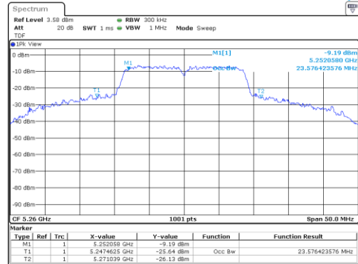
UNII-2A / 802.11n(HT20) / 5 260 MHz
