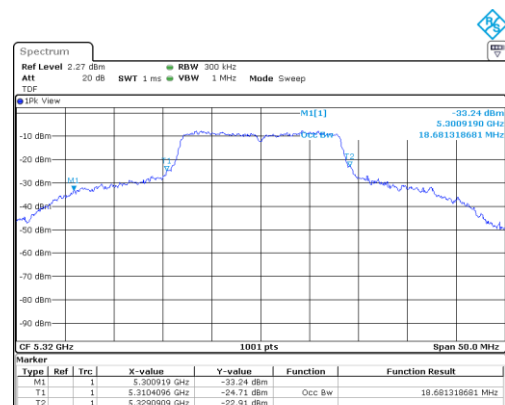
UNII-2A / 802.11a / 5 320 MHz
