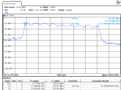
UNII-3 / 802.11ac(VHT80)/ 5 775 MHz
