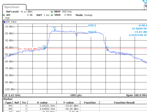
UNII-2C / 802.11ac(VHT40)/ 5 670 MHz
