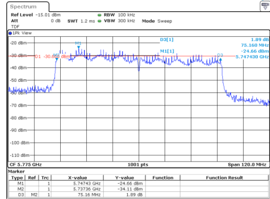
UNII-3 / 802.11ac(VHT80) / 5 775 MHz
