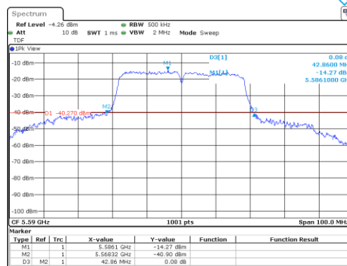
UNII-2C / 802.11ac(VHT40)/ 5 590 MHz
