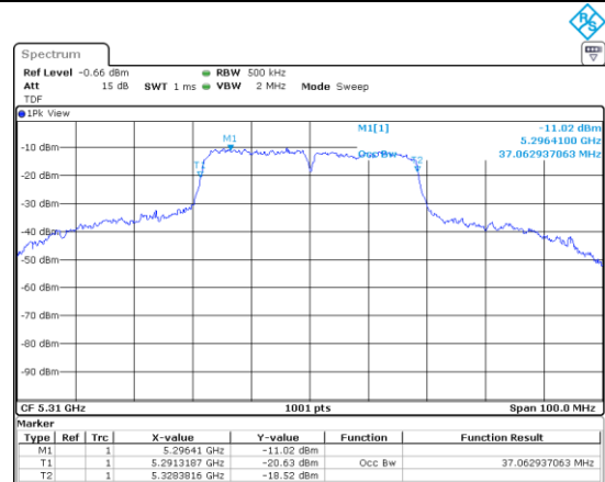
UNII-2A / 802.ac(VHT40)/ 5 310 MHz
