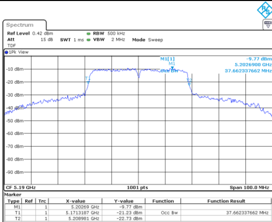
UNII-1 / 802.ac(VHT40)/ 5 190 MHz
