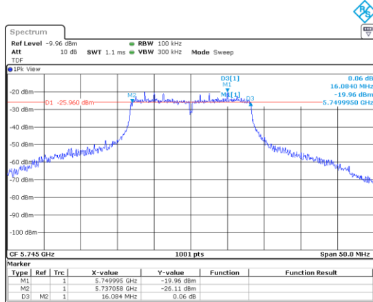
UNII-3 / 802.11a / 5 745 MHz
