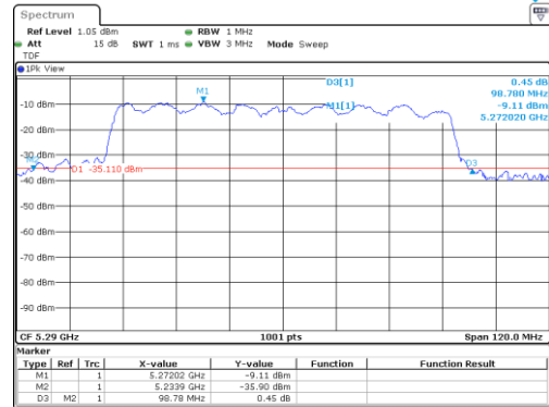
UNII-2A / 802.11ac(VHT80)/ 5 290 MHz
