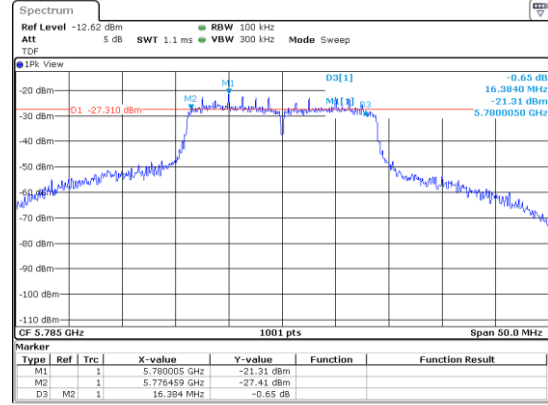
UNII-3 / 802.11n(HT20) / 5 785 MHz
