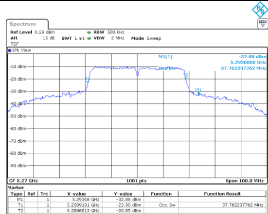
UNII-2A / 802.ac(VHT40)/ 5 270 MHz
