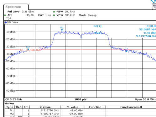
UNII-2A / 802.11n(HT20) / 5 320 MHz
