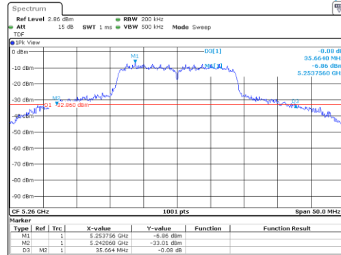
UNII-2A / 802.11n(HT20) / 5 260 MHz
