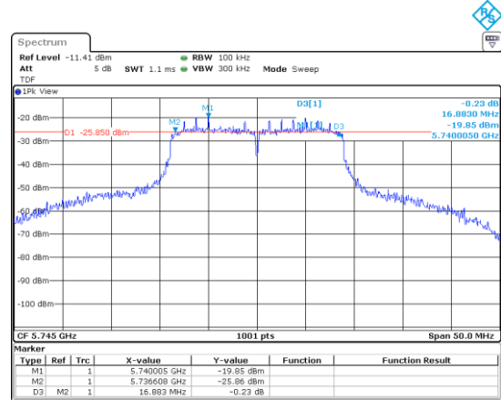
UNII-3 / 802.11n(HT20) / 5 745 MHz
