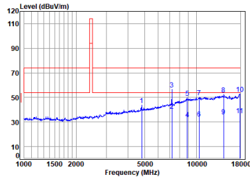
2.4G_SRD_TX_LOW_Horizontal
