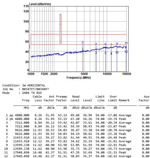
2.4G_SRD_LOW_TX_Horizontal
