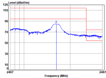
MIN-1050 2.4G SRD_TX_CH_H_Horizontal
