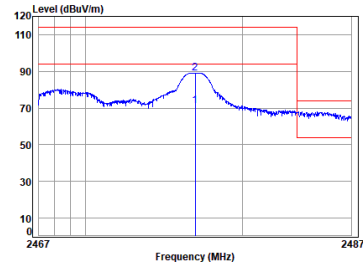
MIN-1050 2.4G SRD_TX_CH_H_Vertical
