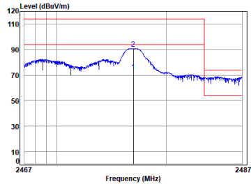
MIN-1052 2.4G SRD_TX_CH_H_Horizontal
