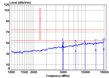
MIN-1052 2.4G SRD_TX_CH_H_Vertical
