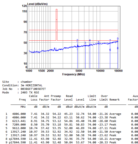
MIN-1052 2.4G SRD_TX_CH_L_Horizontal
