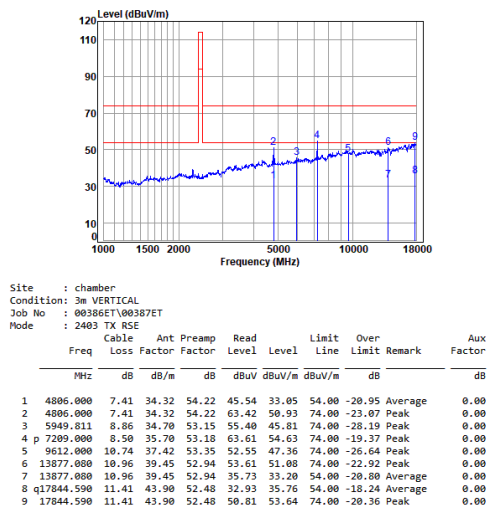
MIN-1052 2.4G SRD_TX_CH_L_Vertical
